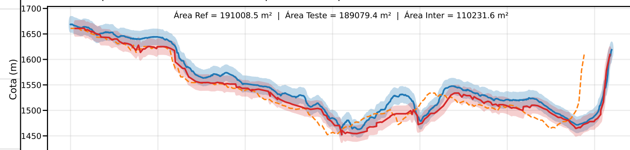
Classe D | PEC-PCD (Vertical)=15.0 m | EQ = 20m | dm = 20.13
