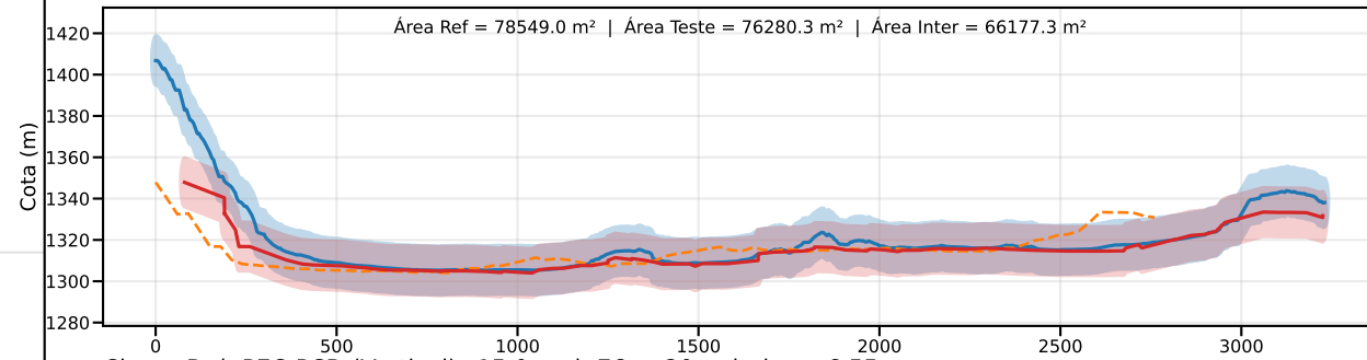
Classe D | PEC-PCD (Vertical)=15.0 m | EQ = 20m | dm = 6.55
