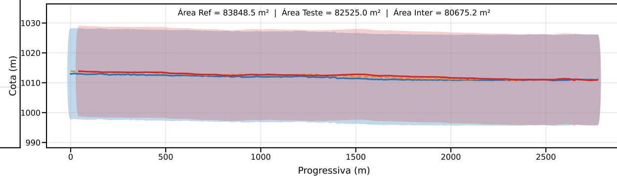
Classe D | PEC-PCD (Vertical)=15.0 m | EQ = 20m | dm = 1.81
