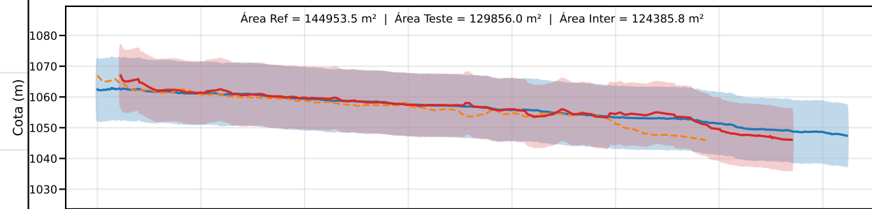
Classe C | PEC-PCD (Vertical)=12.0 m | EQ = 20m | dm = 5.70
