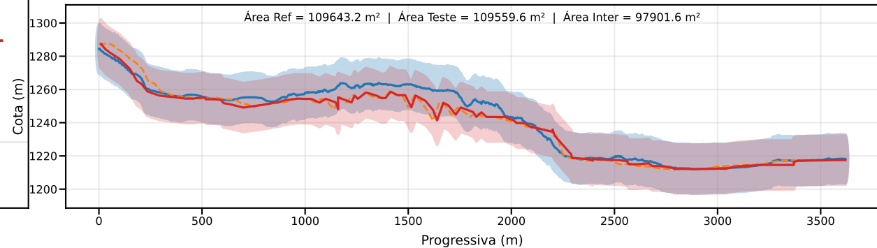
Classe D | PEC-PCD (Vertical)=15.0 m | EQ = 20m | dm = 5.05
