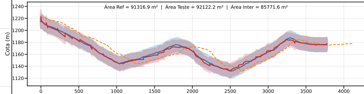
Classe D | PEC-PCD (Vertical)=15.0 m | EQ = 20m | dm = 2.26
