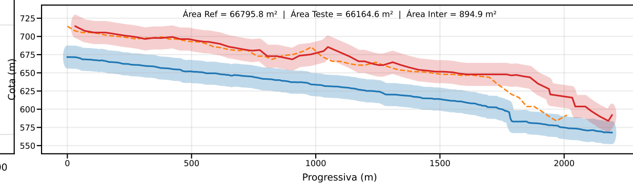
Classe D | PEC-PCD (Vertical)=15.0 m | EQ = 20m | dm = 46.94
