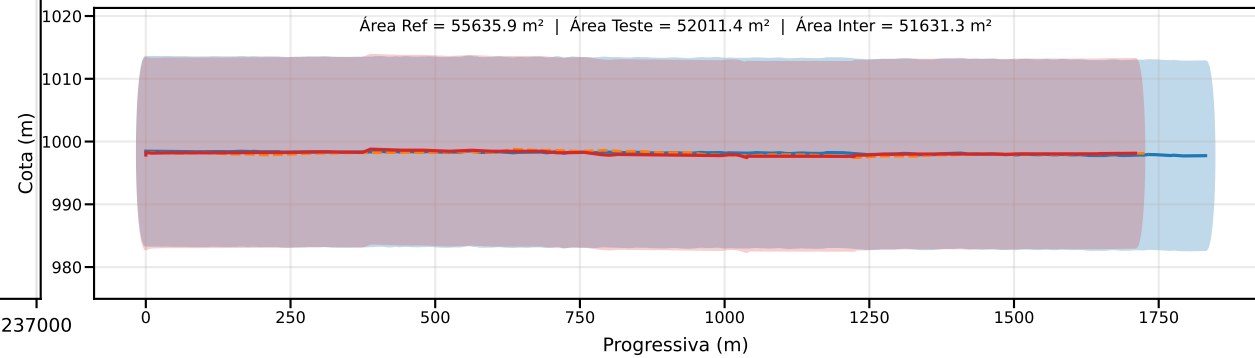
Classe D | PEC-PCD (Vertical)=15.0 m | EQ = 20m | dm = 3.63
