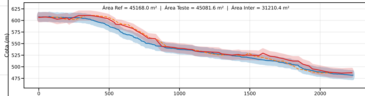
Classe C | PEC-PCD (Vertical)=12.0 m | EQ = 20m | dm = 9.73
