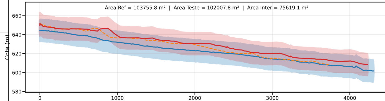
Classe D | PEC-PCD (Vertical)=15.0 m | EQ = 20m | dm = 10.56
