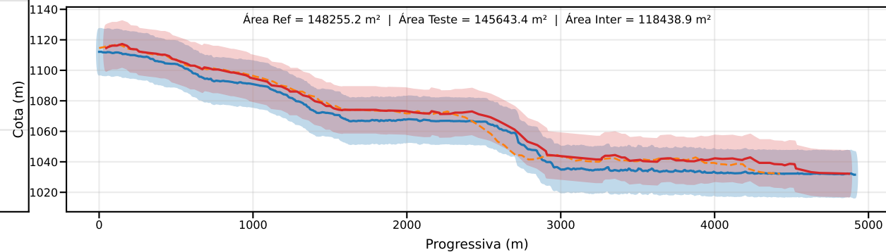
Classe D | PEC-PCD (Vertical)=15.0 m | EQ = 20m | dm = 9.65
