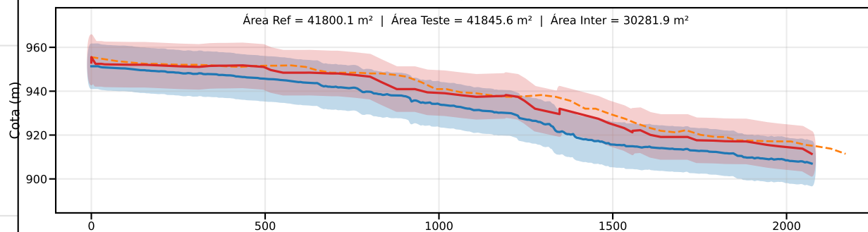
Classe C | PEC-PCD (Vertical)=12.0 m | EQ = 20m | dm = 8.64
