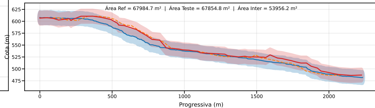
Classe D | PEC-PCD (Vertical)=15.0 m | EQ = 20m | dm = 9.74
