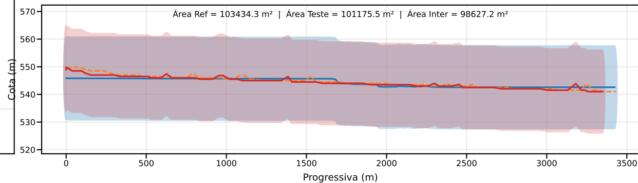
Classe D | PEC-PCD (Vertical)=15.0 m | EQ = 20m | dm = 2.24
