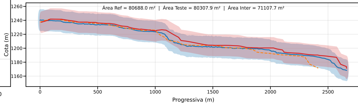
Classe D | PEC-PCD (Vertical)=15.0 m | EQ = 20m | dm = 5.62
