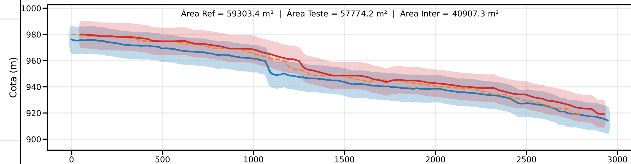
Classe C | PEC-PCD (Vertical)=12.0 m | EQ = 20m | dm = 10.16
