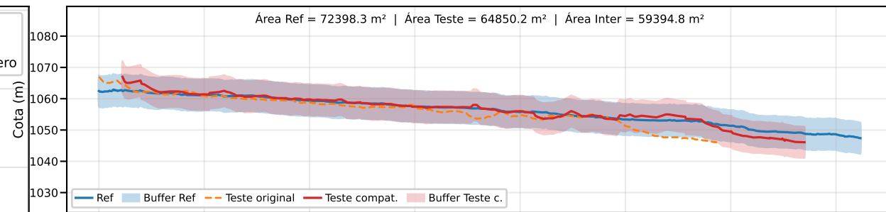
Classe B | PEC-PCD (Vertical)=10.0 m | EQ = 20m | dm = 4.98
