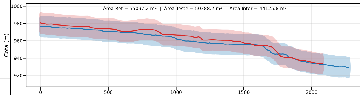
Classe D | PEC-PCD (Vertical)=15.0 m | EQ = 20m | dm = 9.08
