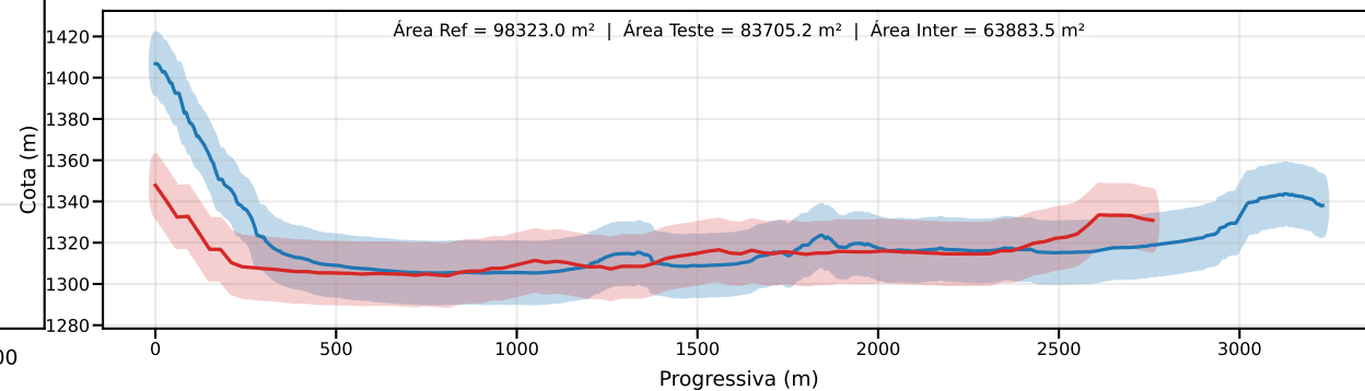
Classe D | PEC-PCD (Vertical)=15.0 m | EQ = 20m | dm = 19.39
