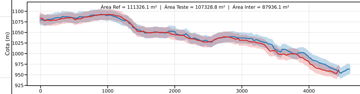
Classe D | PEC-PCD (Vertical)=15.0 m | EQ = 20m | dm = 8.56
