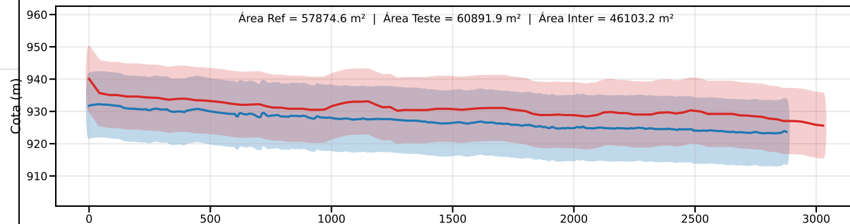
Classe C | PEC-PCD (Vertical)=12.0 m | EQ = 20m | dm = 6.08
