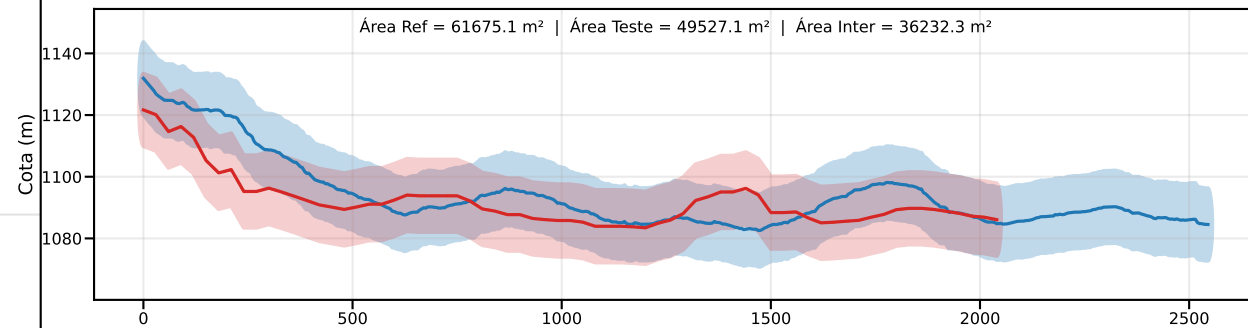
Classe D | PEC-PCD (Vertical)=15.0 m | EQ = 20m | dm = 21.65
