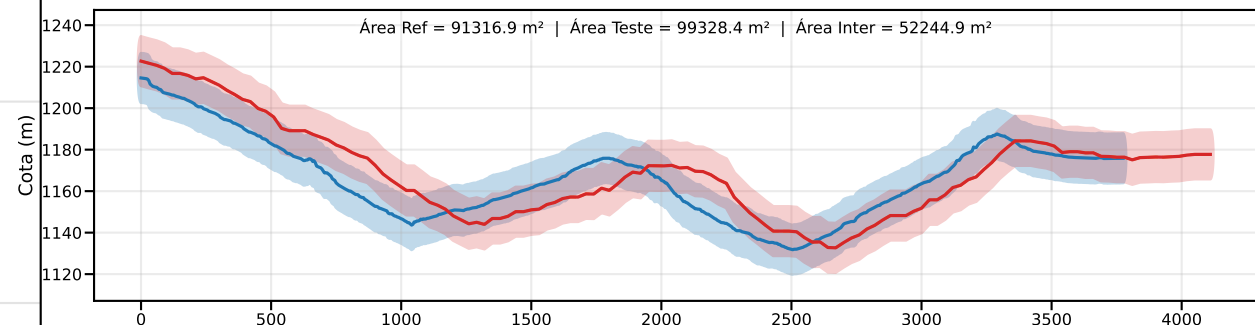
Classe D | PEC-PCD (Vertical)=15.0 m | EQ = 20m | dm = 14.82
