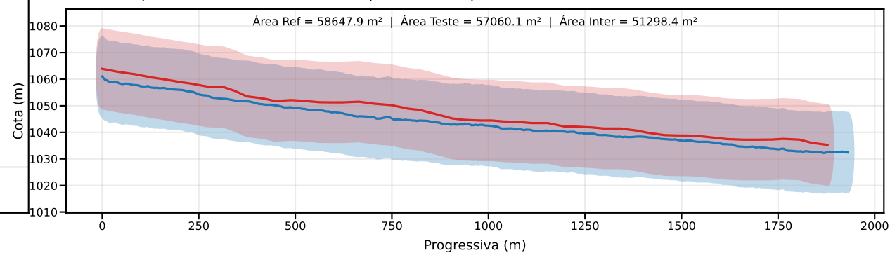
Classe D | PEC-PCD (Vertical)=15.0 m | EQ = 20m | dm = 6.07
