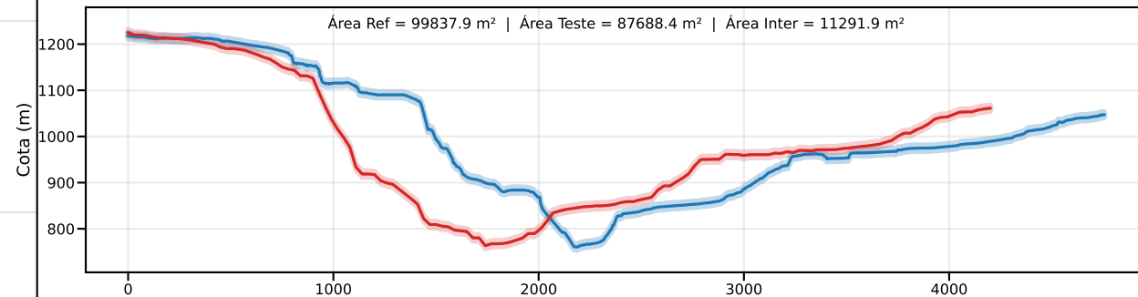
Classe C | PEC-PCD (Vertical)=12.0 m | EQ = 20m | dm = 37.05
