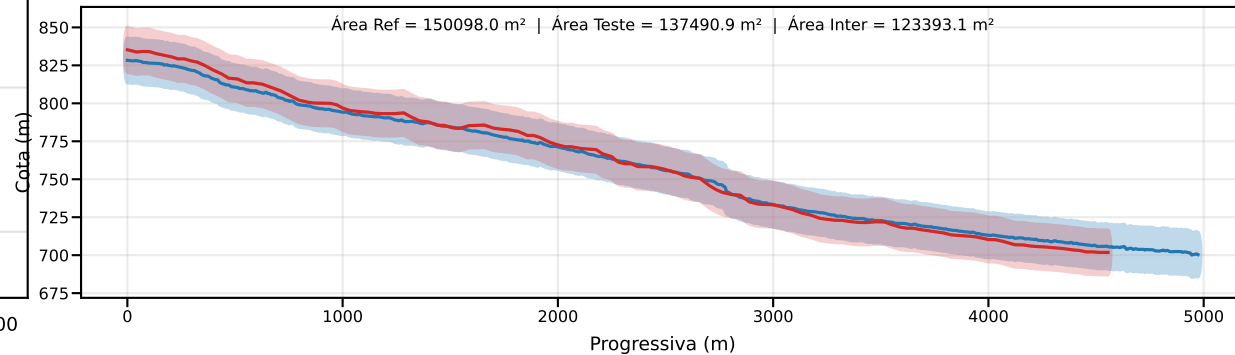
Classe D | PEC-PCD (Vertical)=15.0 m | EQ = 20m | dm = 9.15
