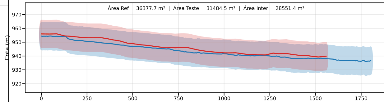
Classe C | PEC-PCD (Vertical)=12.0 m | EQ = 20m | dm = 8.77
