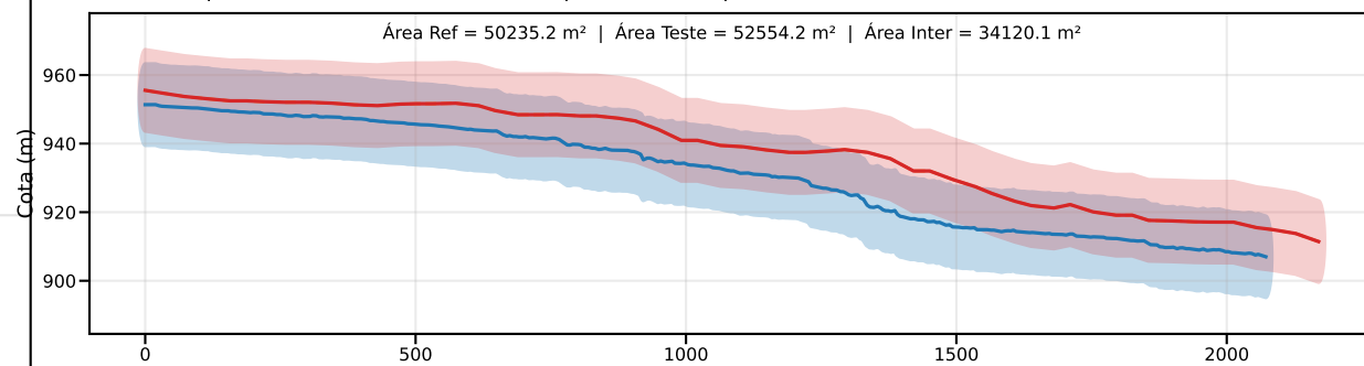
Classe D | PEC-PCD (Vertical)=15.0 m | EQ = 20m | dm = 11.55
