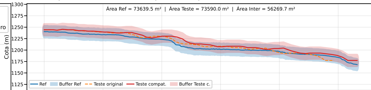
Classe B | PEC-PCD (Vertical)=25.0 m | EQ = 50m | dm = 10.19
