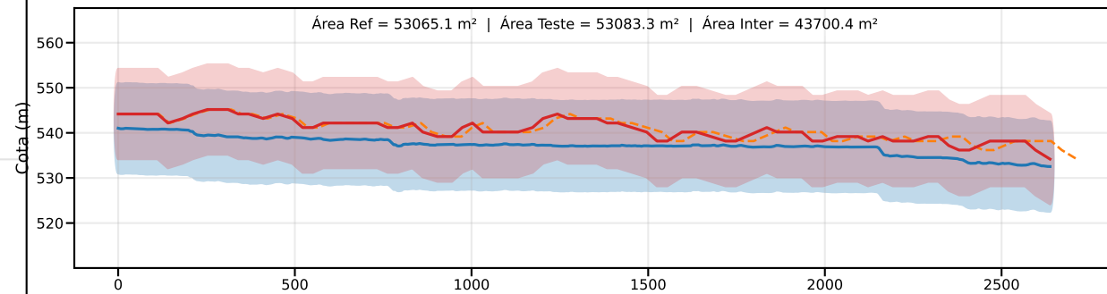
Classe C | PEC-PCD (Vertical)=12.0 m | EQ = 20m | dm = 5.54
