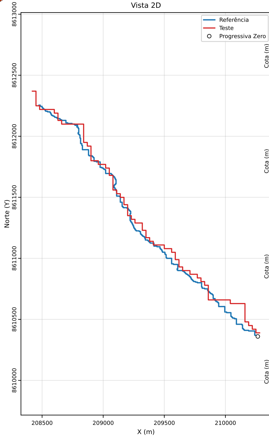
Classe A | PEC-PCD (Vertical)=27.0 m | EQ = 100m | dm = 3.01
