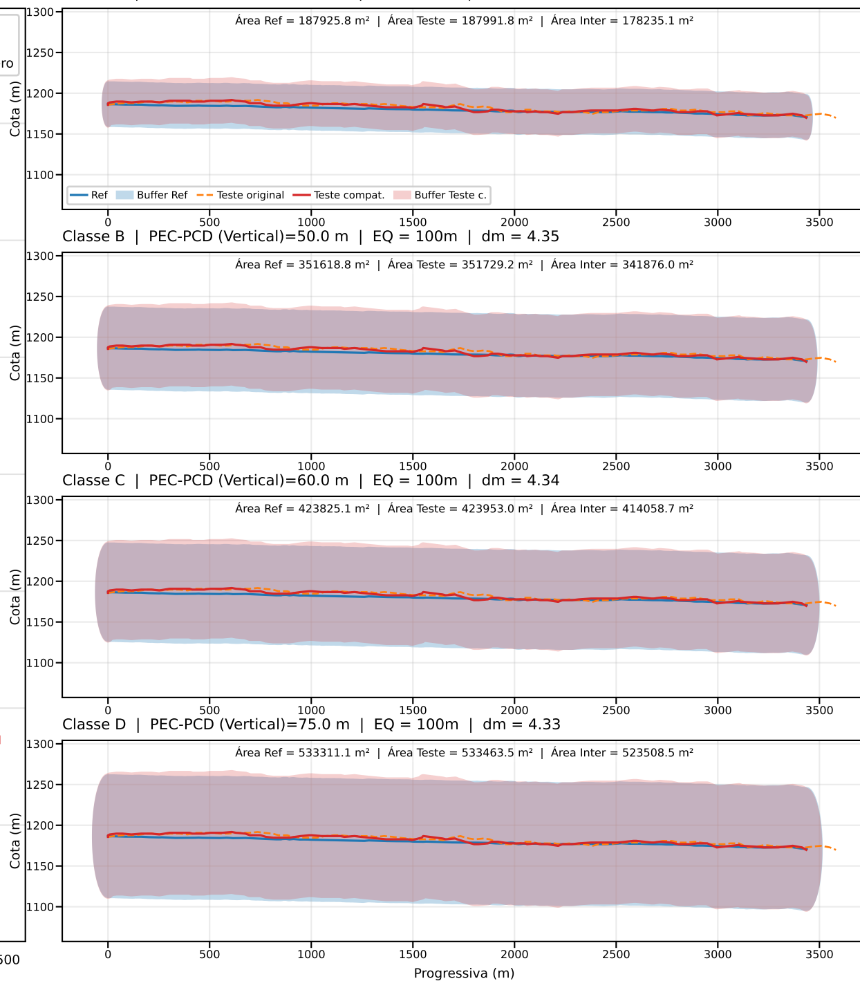
Classe A | PEC-PCD (Vertical)=27.0 m | EQ = 100m | dm = 4.37
