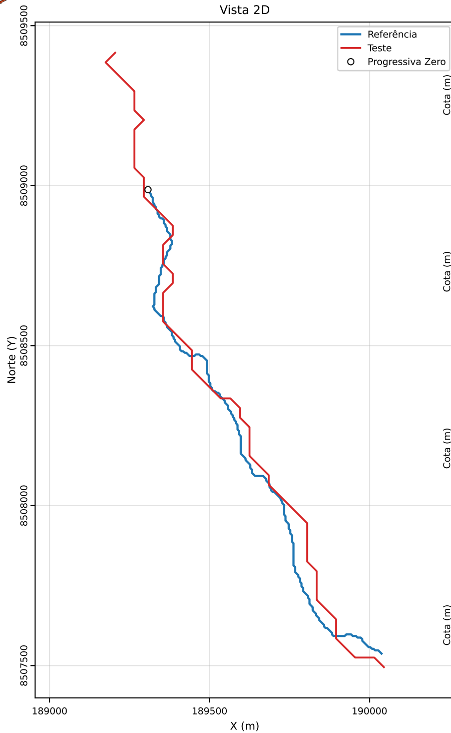
Classe A | PEC-PCD (Vertical)=27.0 m | EQ = 100m | dm = 9.48
