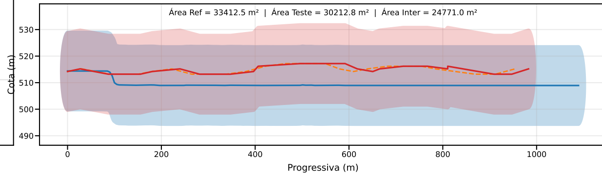
Classe D | PEC-PCD (Vertical)=15.0 m | EQ = 20m | dm = 13.48
