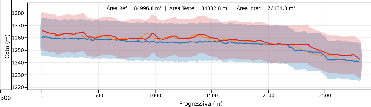
Classe D | PEC-PCD (Vertical)=15.0 m | EQ = 20m | dm = 4.92
