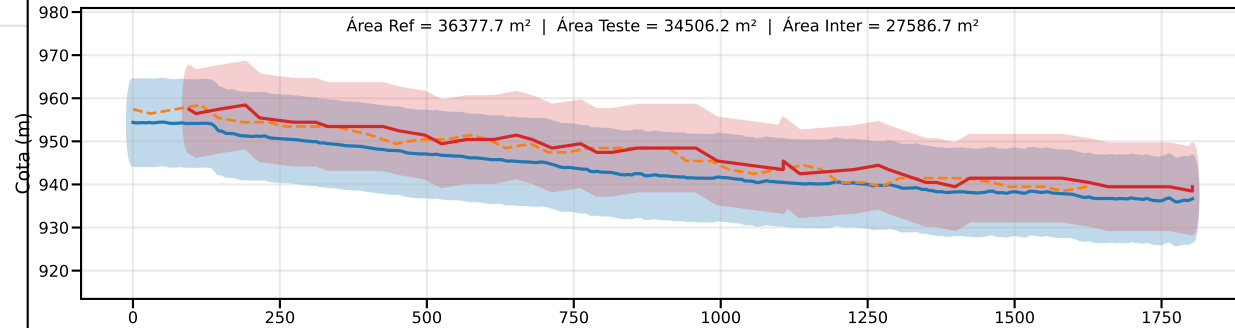
Classe C | PEC-PCD (Vertical)=12.0 m | EQ = 20m | dm = 8.34
