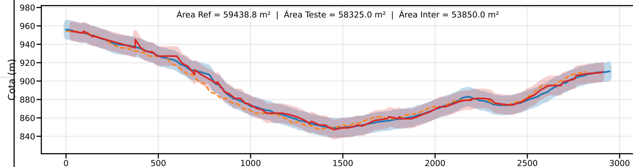
Classe C | PEC-PCD (Vertical)=12.0 m | EQ = 20m | dm = 3.15
