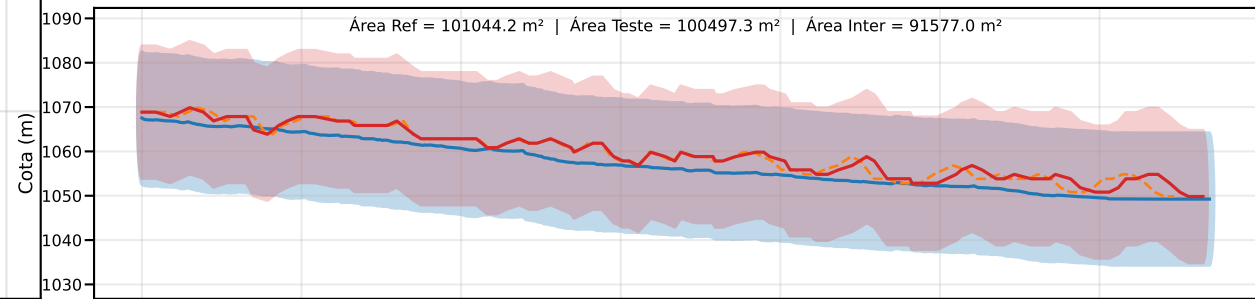
Classe D | PEC-PCD (Vertical)=15.0 m | EQ = 20m | dm = 4.44
