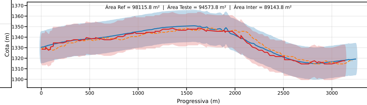
Classe D | PEC-PCD (Vertical)=15.0 m | EQ = 20m | dm = 4.47
