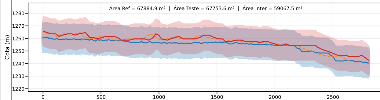
Classe D | PEC-PCD (Vertical)=15.0 m | EQ = 20m | dm = 4.92
