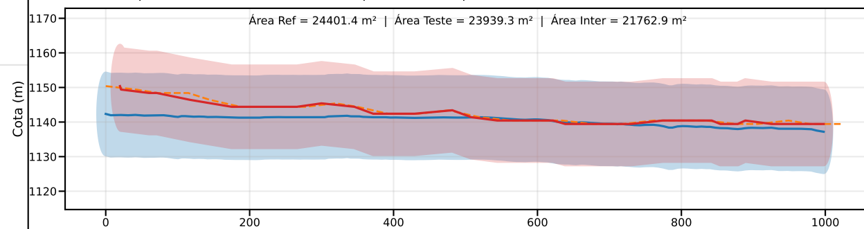
Classe D | PEC-PCD (Vertical)=15.0 m | EQ = 20m | dm = 4.35
