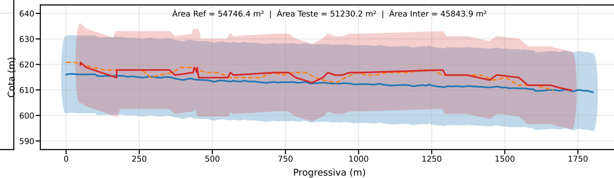
Classe D | PEC-PCD (Vertical)=15.0 m | EQ = 20m | dm = 8.19
