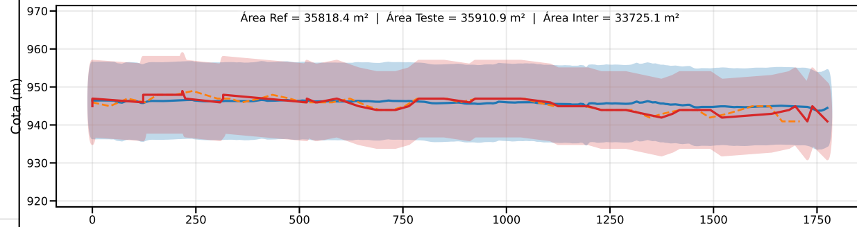
Classe C | PEC-PCD (Vertical)=12.0 m | EQ = 20m | dm = 1.83
