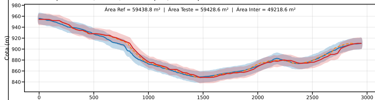
Classe C | PEC-PCD (Vertical)=12.0 m | EQ = 20m | dm = 5.40
