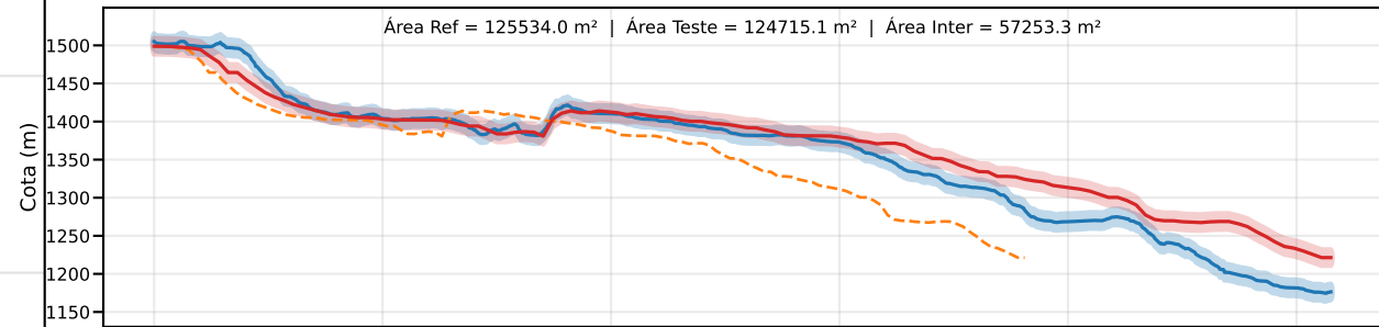
Classe D | PEC-PCD (Vertical)=15.0 m | EQ = 20m | dm = 23.49
