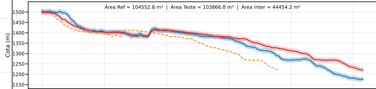
Classe C | PEC-PCD (Vertical)=12.0 m | EQ = 20m | dm = 20.64
