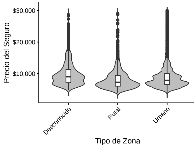
Figure 16: Gráfica de Violín por Zona
