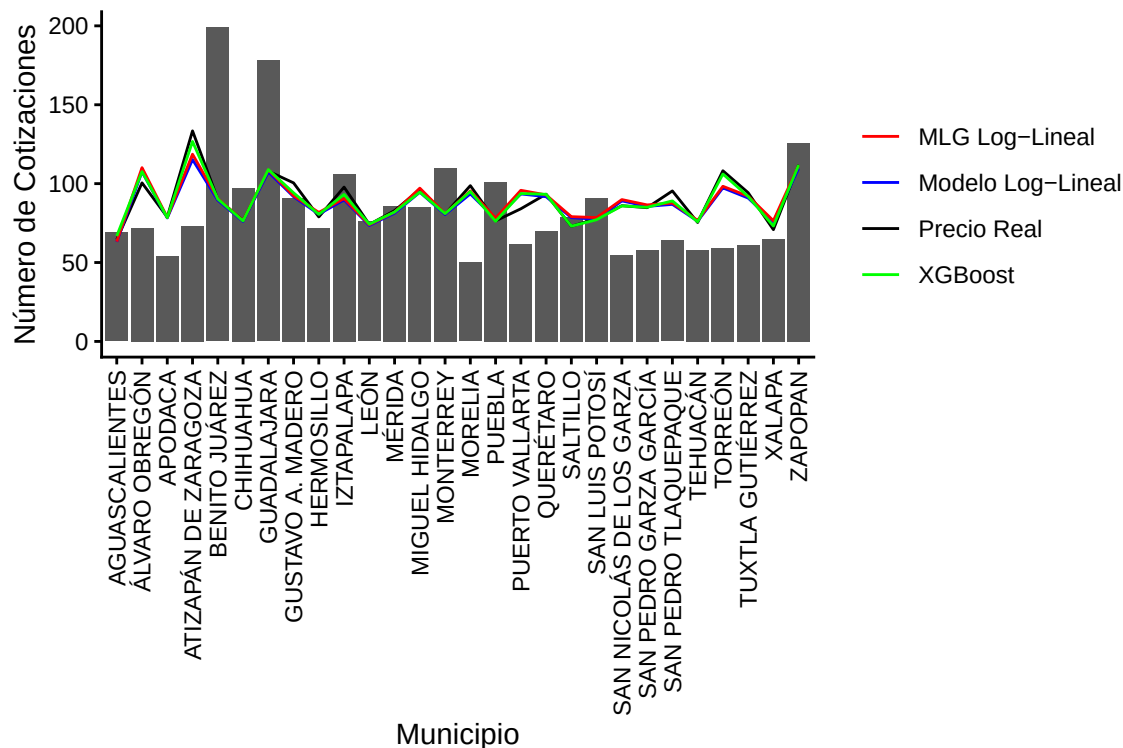
Figure 29: Variable Municipio (mayor a 50 cotizaciones)
