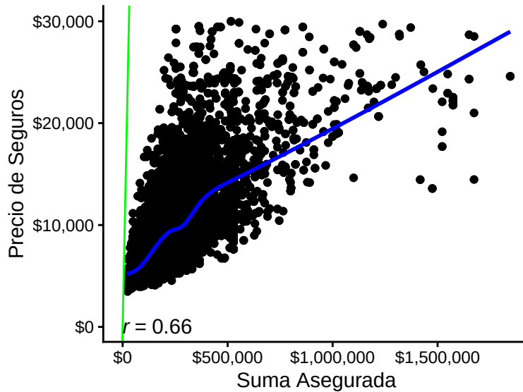
Figure 13: Gráfica de Correlación Precio y Suma Asegurada
