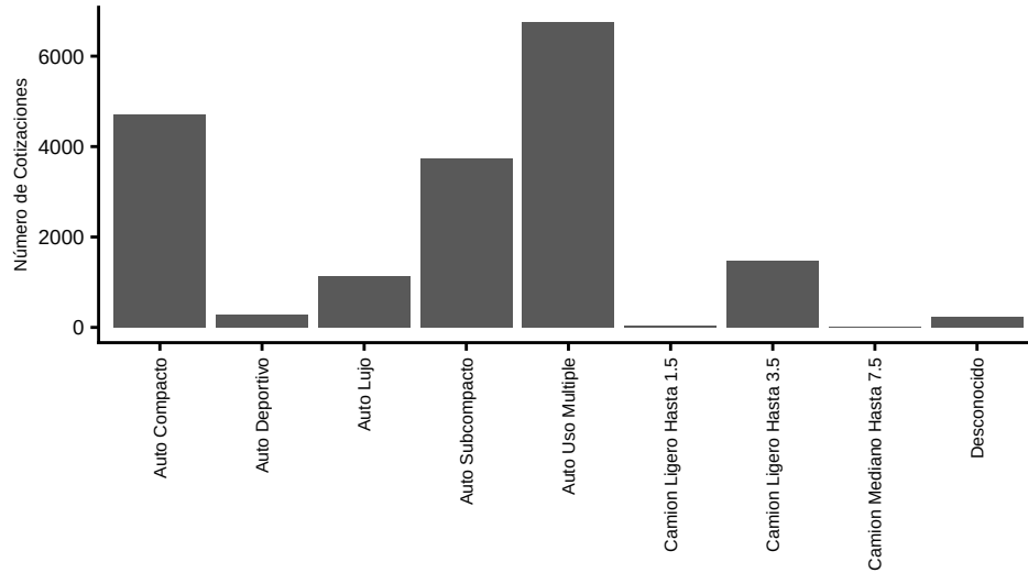
Figure 8: Distribución de la Variable Segmento
