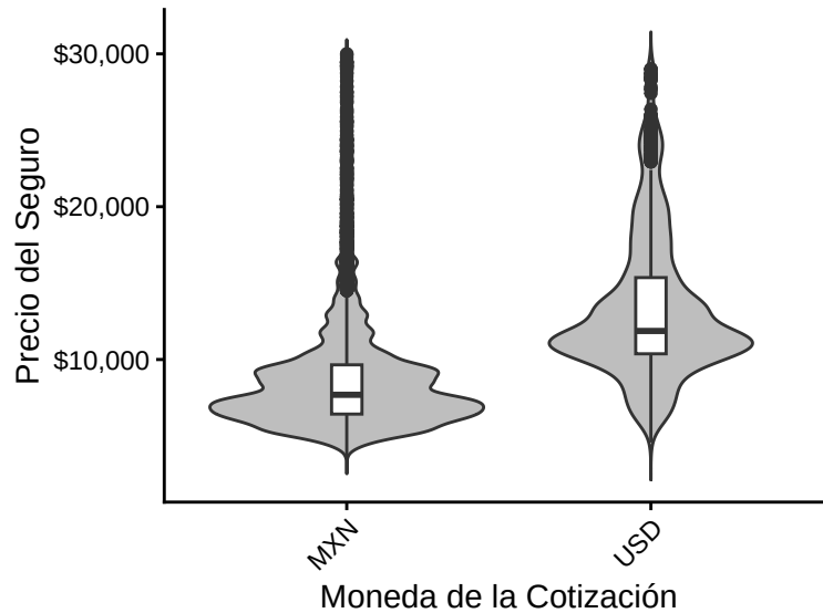
Figure 7: Gráfica de Violín por Moneda
