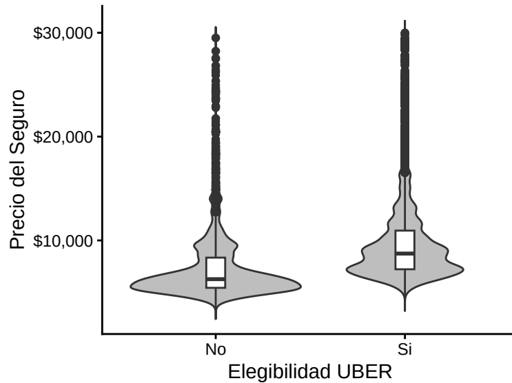
Figure 9: Gráfica de Violín por Elegibilidad de UBER
