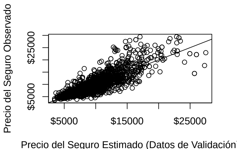
Figure 23: Correlación Valores Reales y Estimados
