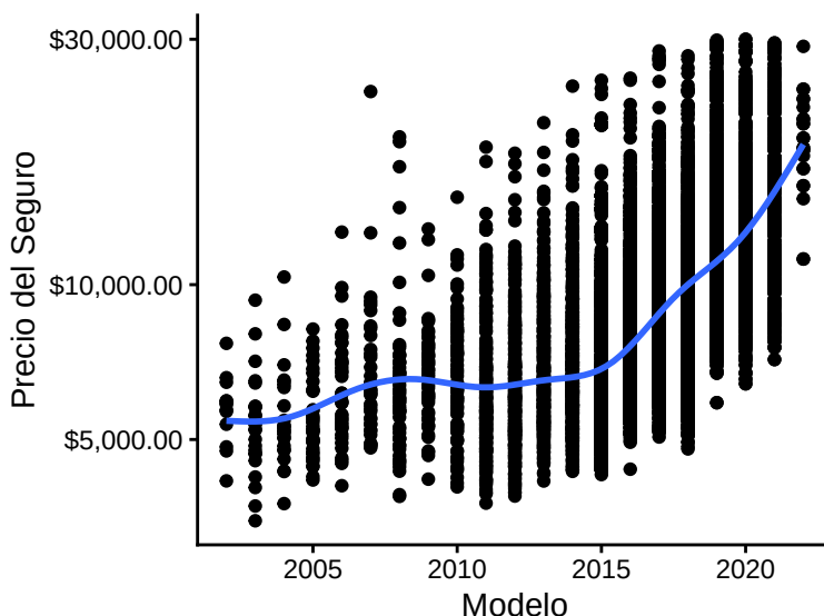
Figure 6: Distribución del Modelo Respecto al Precio
