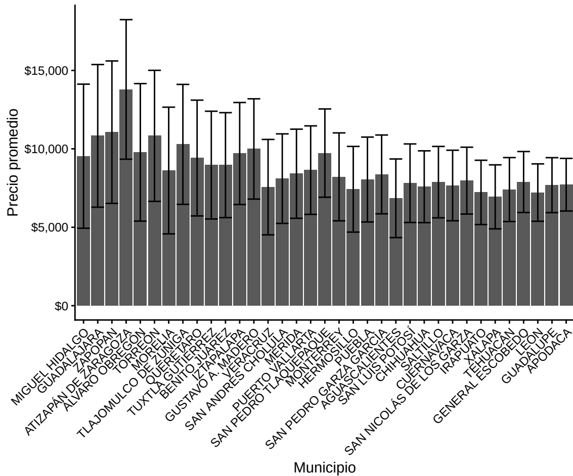
Figure 18: Promedio de Precio por Municipio y su Desviación Estándar
