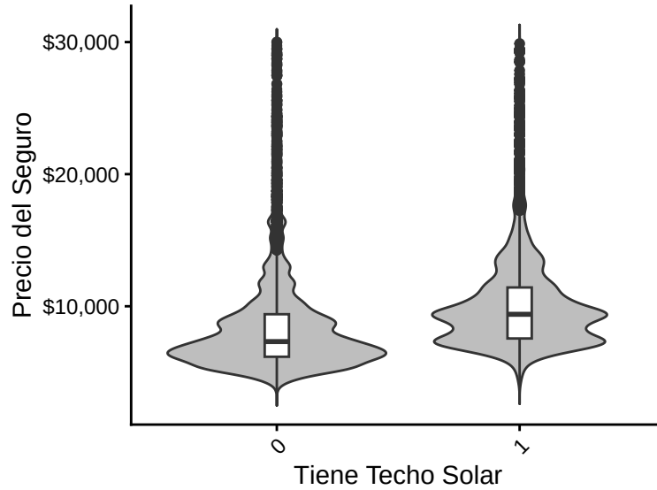
Figure 10: Gráfica de Violín por Techo Solar
