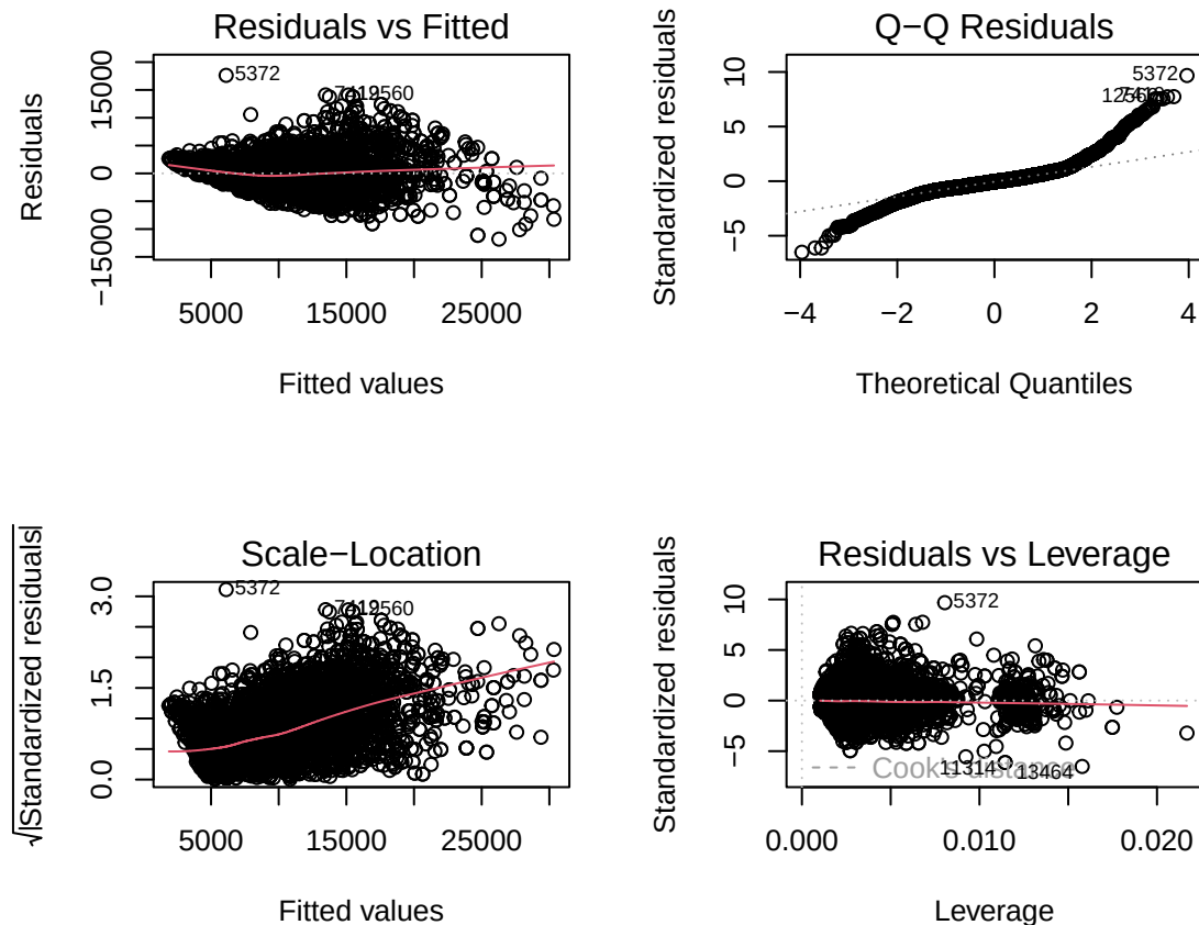
Figure 19: Análisis de Supuestos del Modelo Lineal
