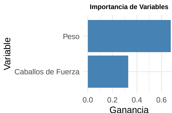
Figure 4: Ejemplo de Importancia de Variables
