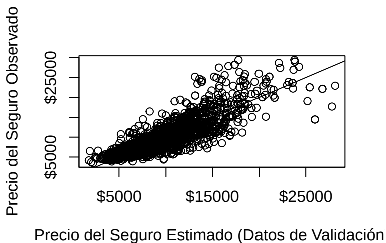
Figure 20: Correlación Valores Reales y Estimados
