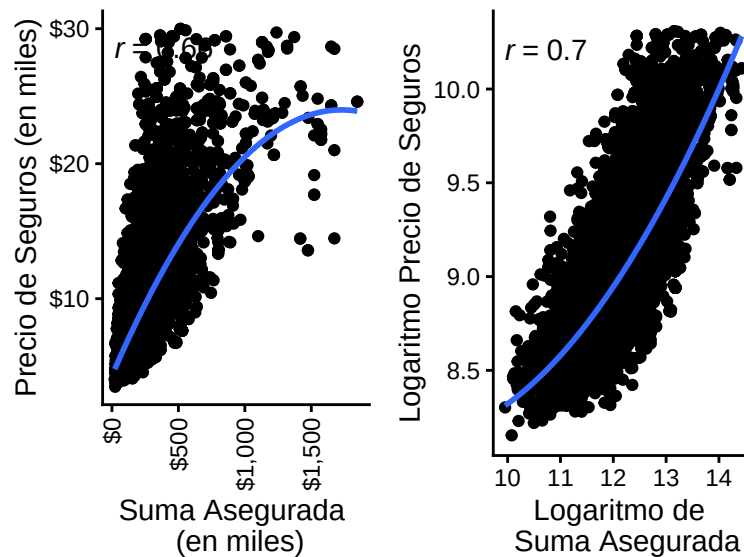
Figure 15: Correlación Suma Asegurada Término Cuadrado y Logarítmico
