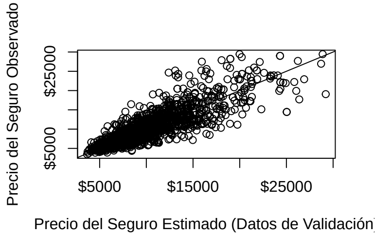
Figure 25: Correlación Valores Reales y Estimados
