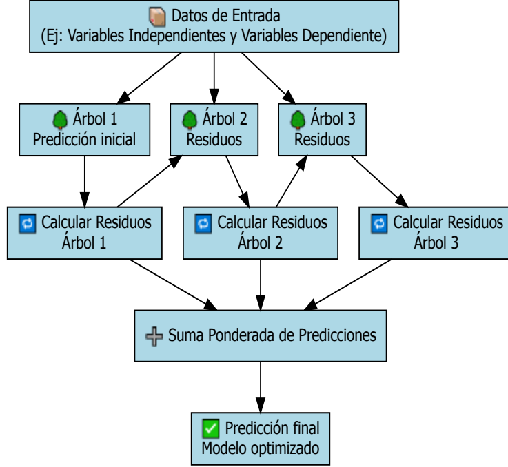
Figure 3: Diagrama de 3 Iteraciones del Algoritmo del Modelo de XGradient Boosting
