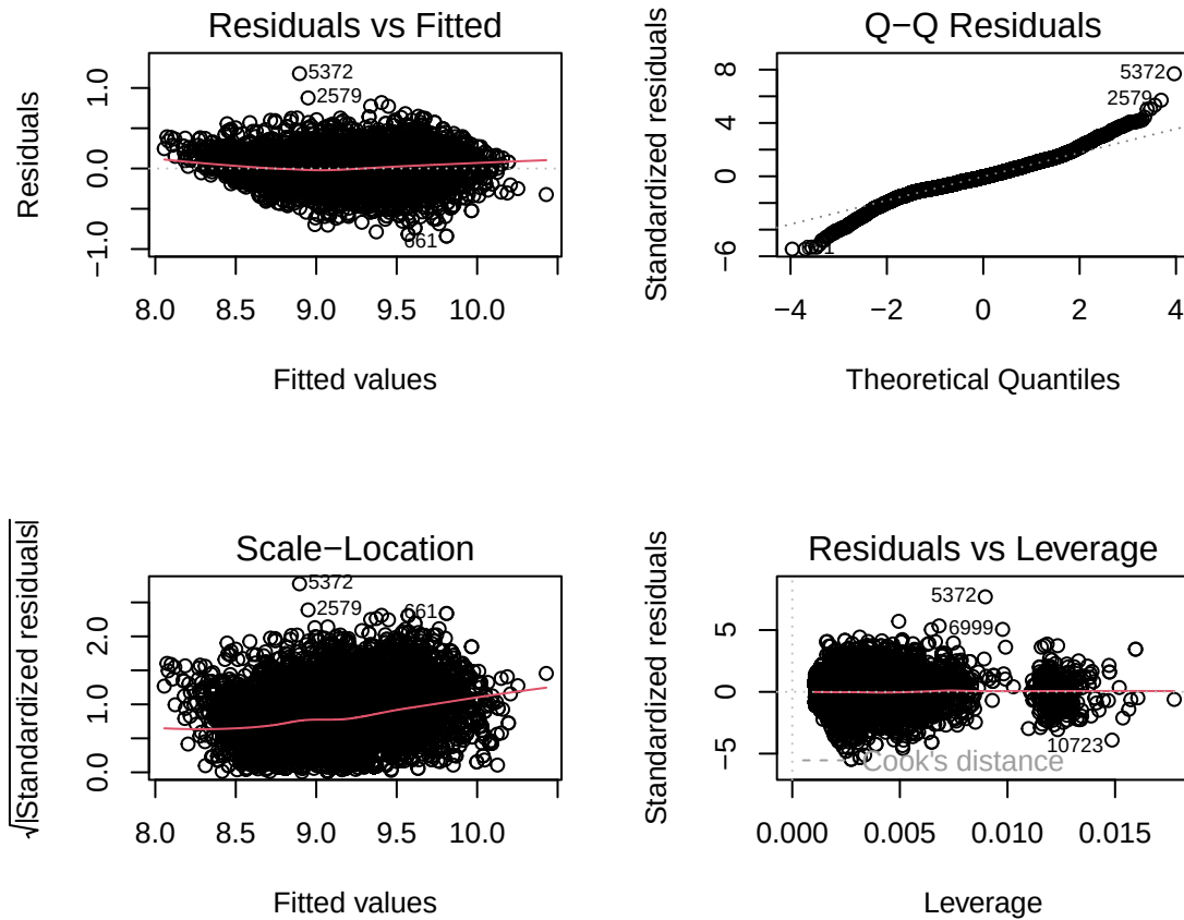
Figure 21: Análisis de Supuestos del Modelo Lineal
