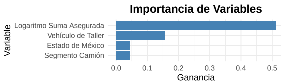
Figure 26: Importancia de las Variables
