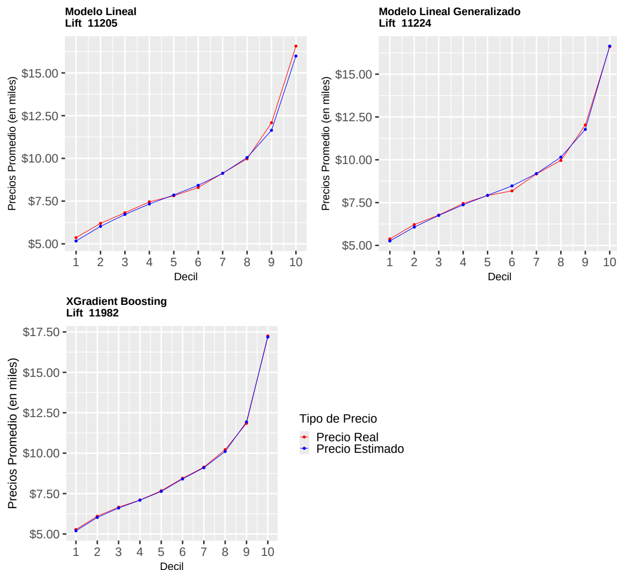
Figure 31: Gráficos de Cuantiles
