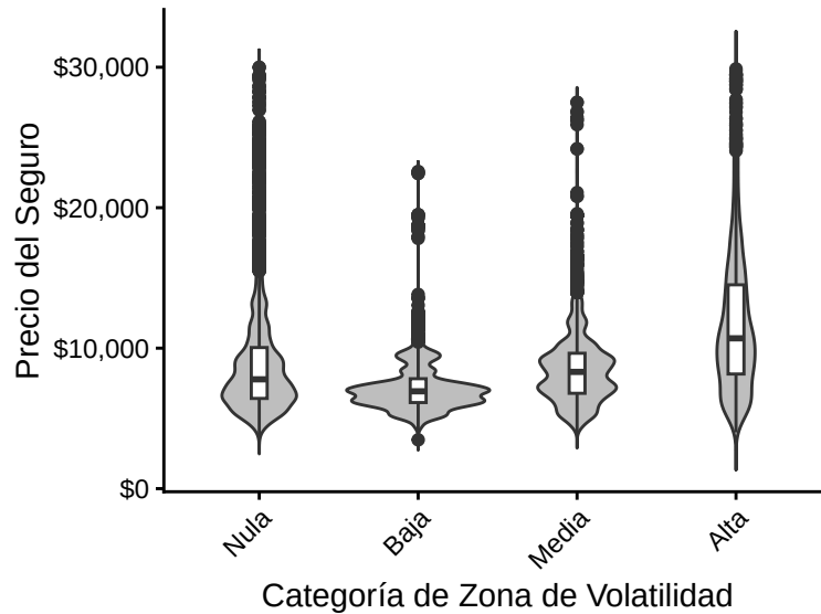
Figure 12: Gráfica de Violín por Zona de Volatilidad
