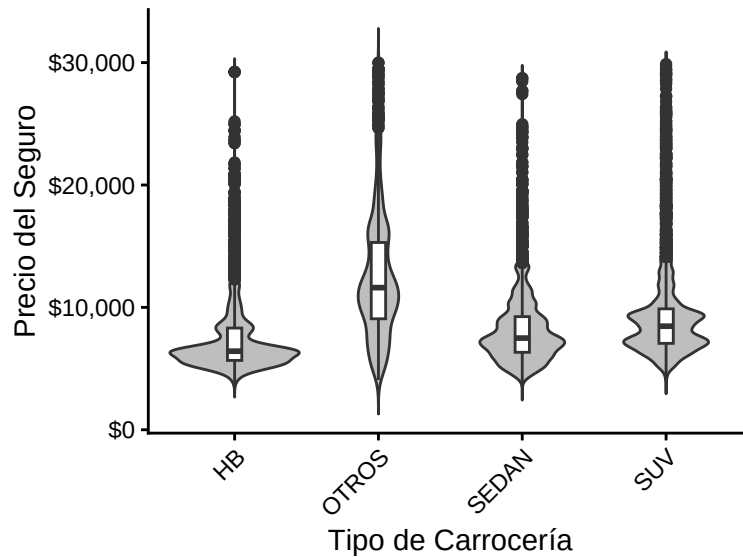
Figure 17: Gráfica de Violín por Carrocería
