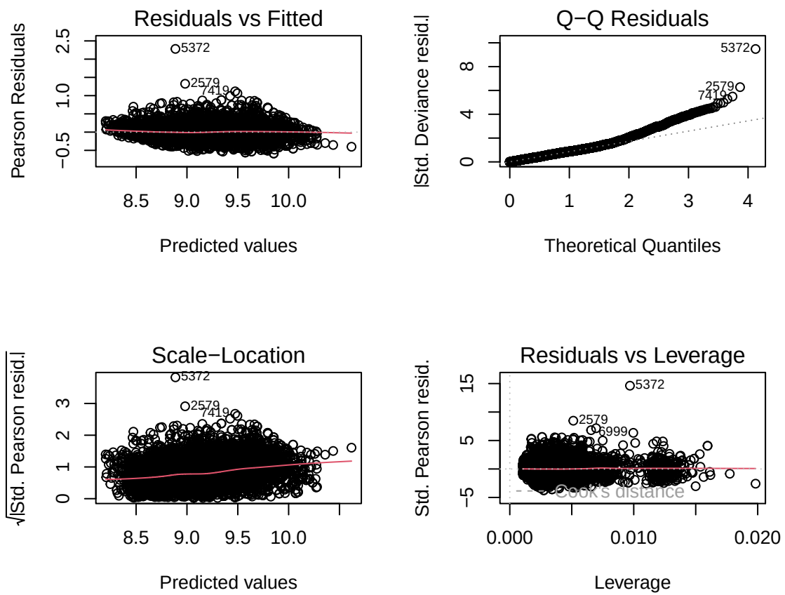
Figure 24: Análisis de al Ajuste del Modelo Lineal Generalizado
