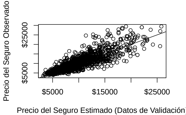
Figure 22: Correlación Valores Reales y Estimados
