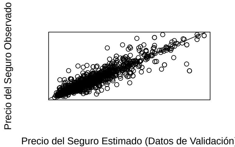
Figure 27: Correlación Valores Reales y Estimados
