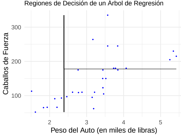
Figure 2: Partición del Espacio de Variables Predictoras
