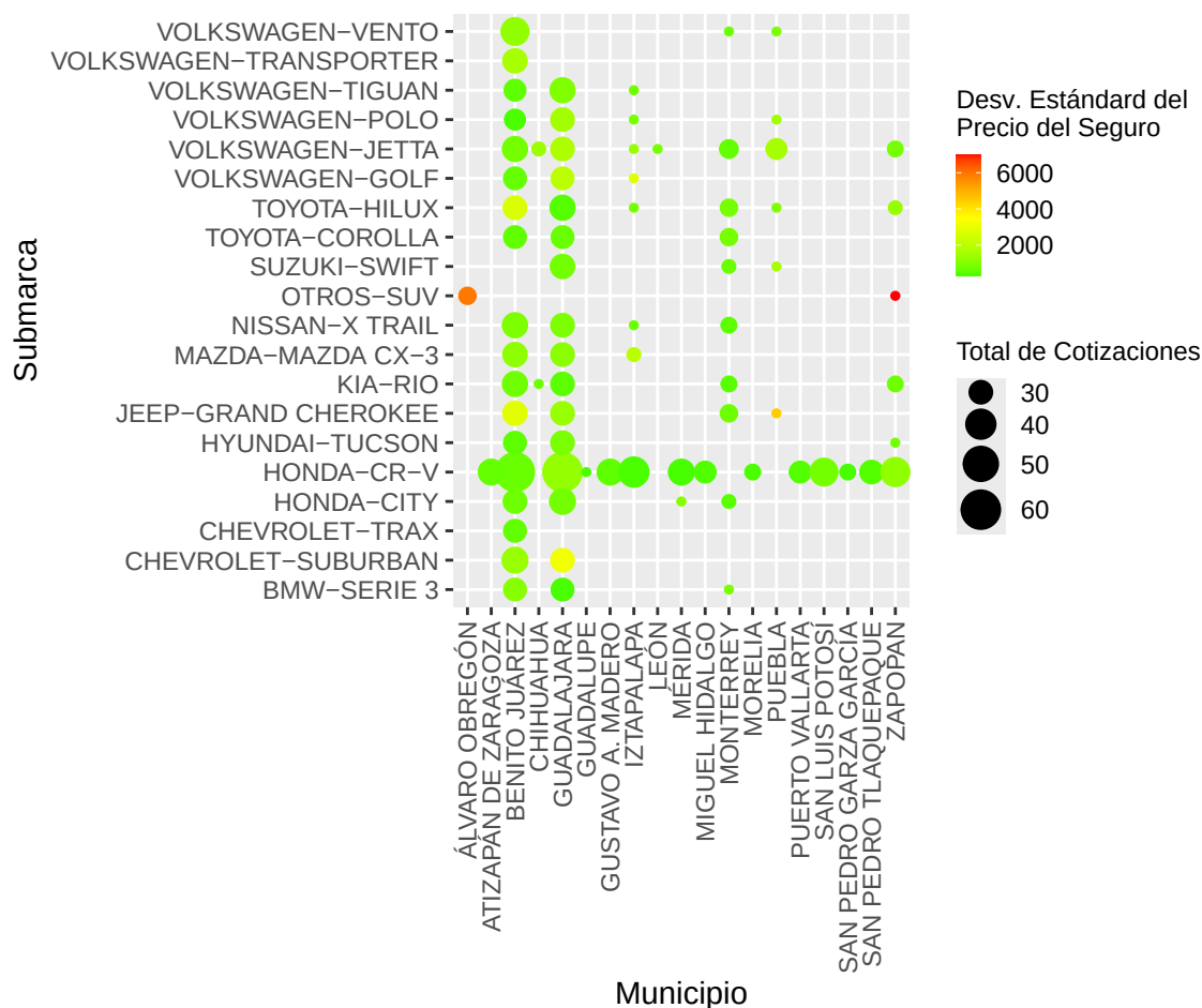
Figure 11: Mapa de Calor por Municipio y Submarca
