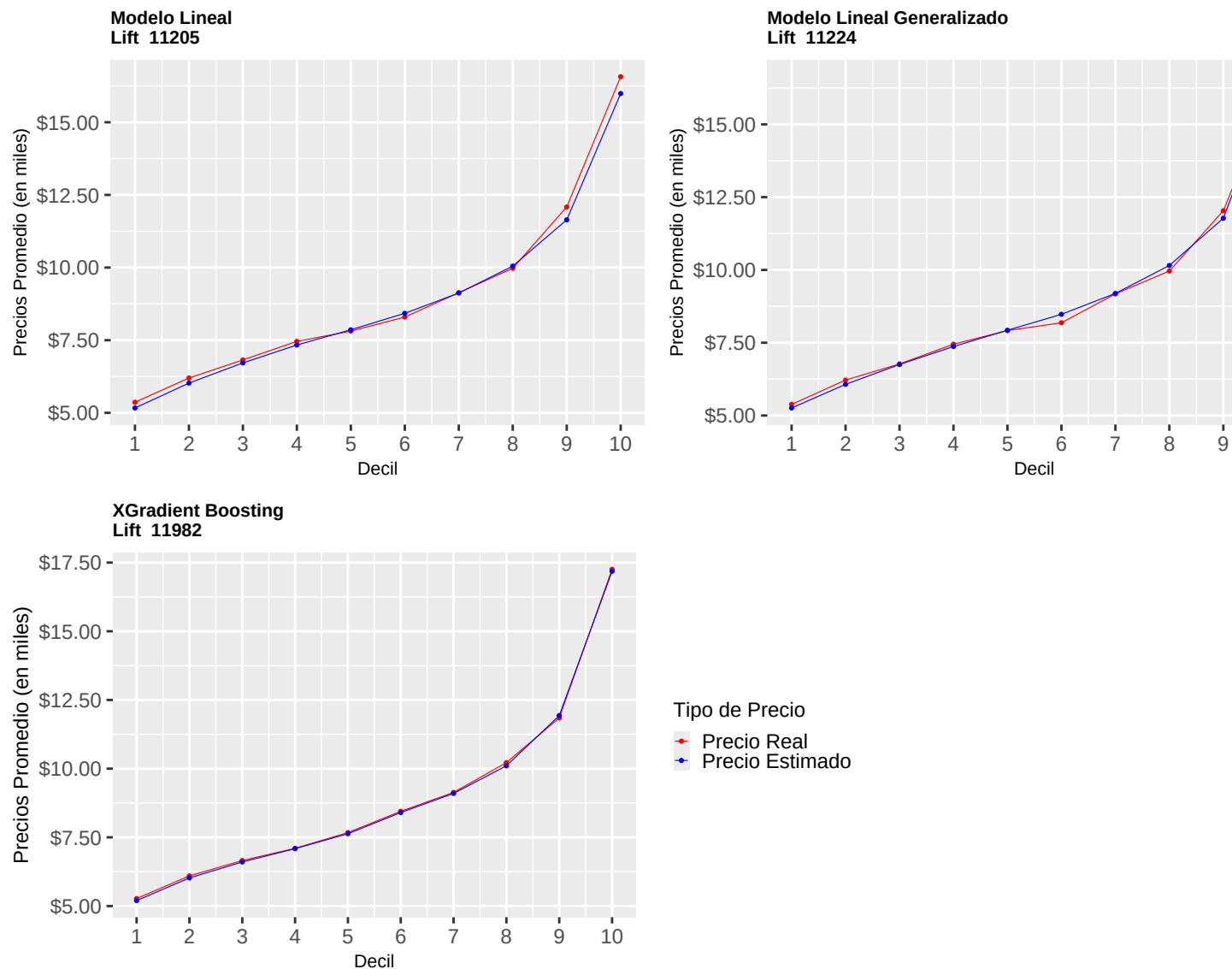
Figura 30: Gráficos de Cuantiles
