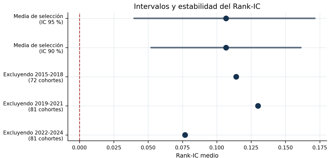
Figura 6.7: Intervalos de confianza del Rank-IC por bloques y estabilidad de la media al excluir cada era completa.
