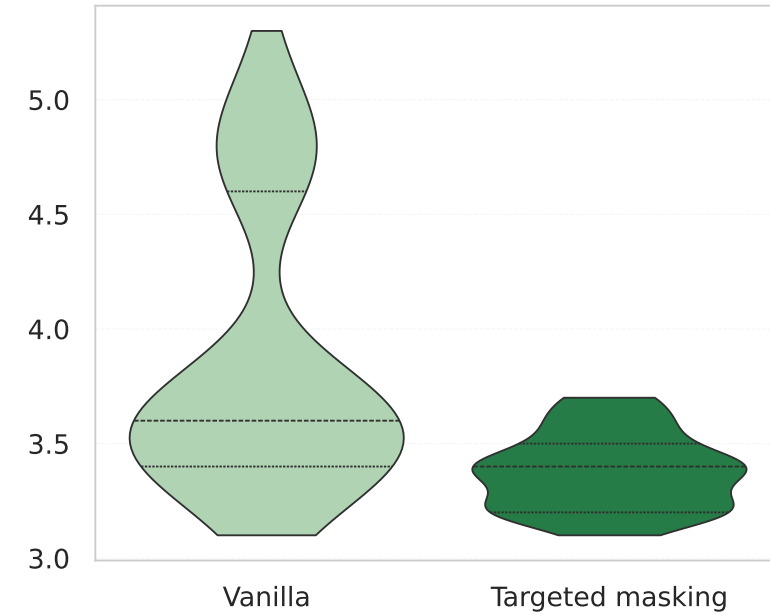
shortest_LYS307D-GLU241D
