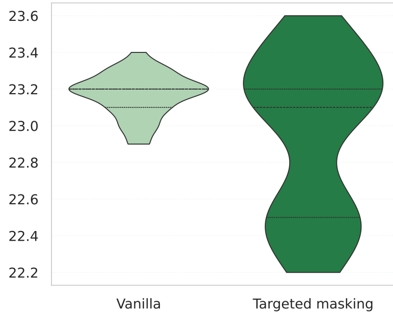
shortest_ARG292B-GLU231B
