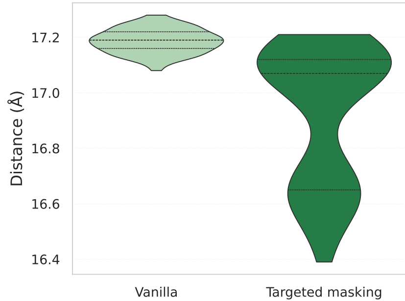
B_ARG298-B_PHE238
