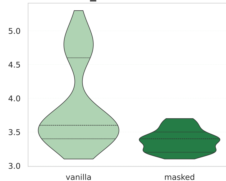
shortest_LYS307D-GLU241D
