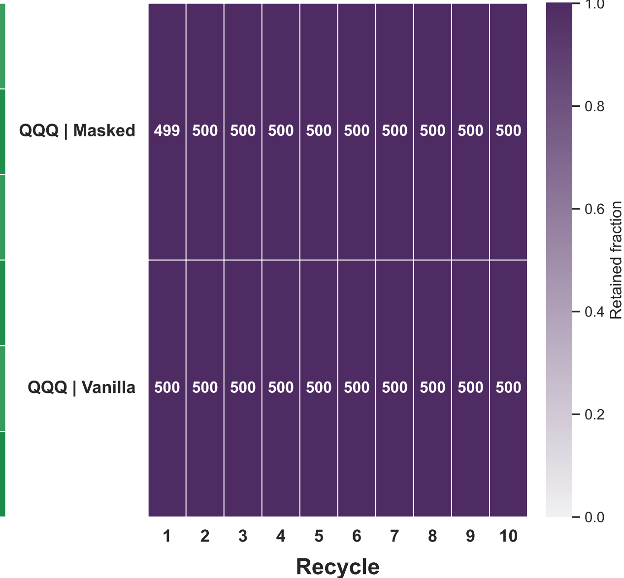
NaV1.5
