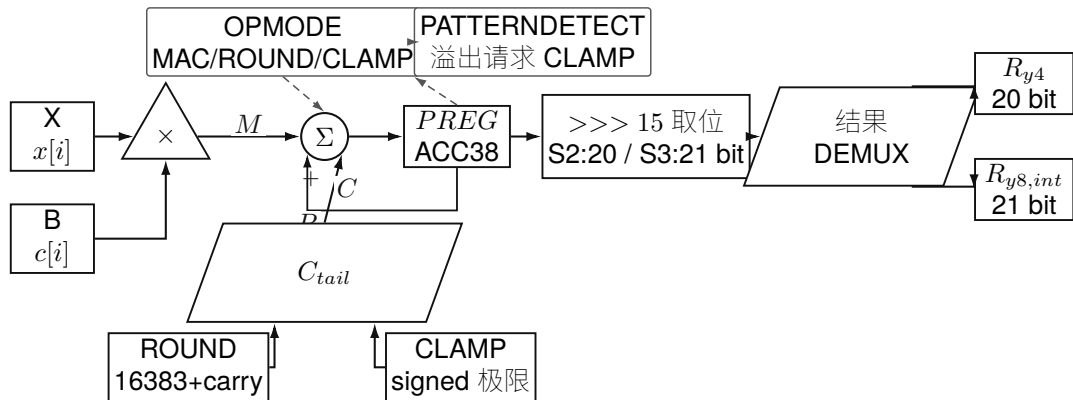
(b) DSP 内 MAC、ROUND 与 CLAMP
