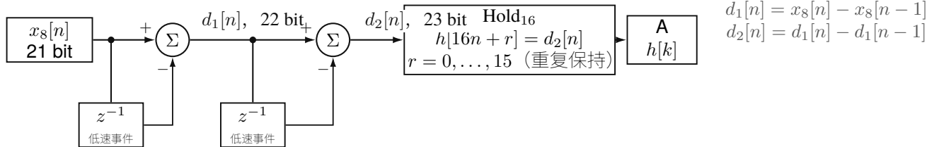
(a) 低速二阶差分与 16 倍保持
