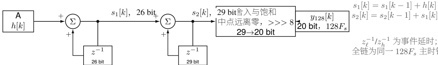
(b) 高速二阶积分与定点输出
