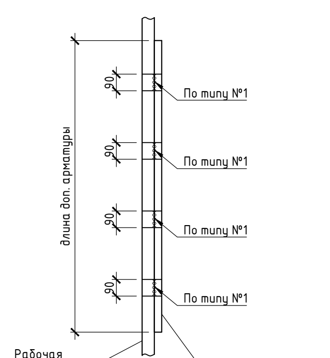
Схема стыковки сабвенной арматуры
