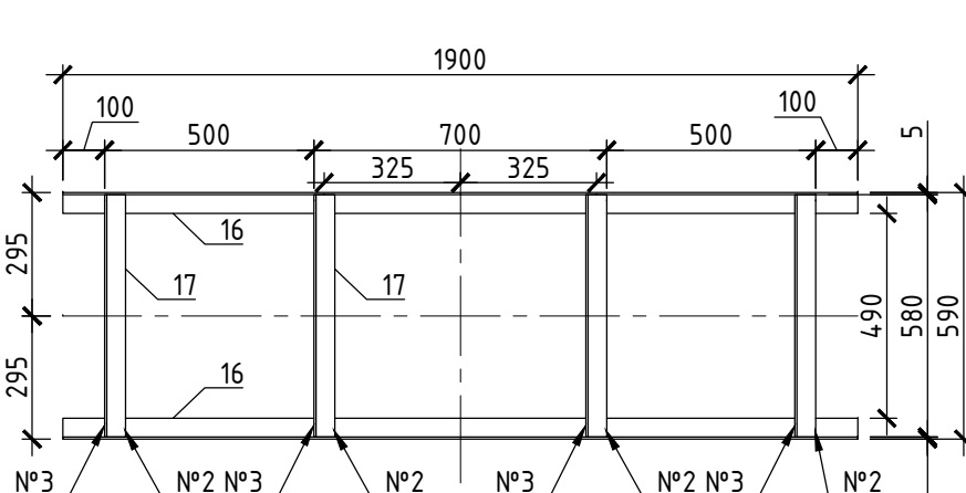
Рама Р15
