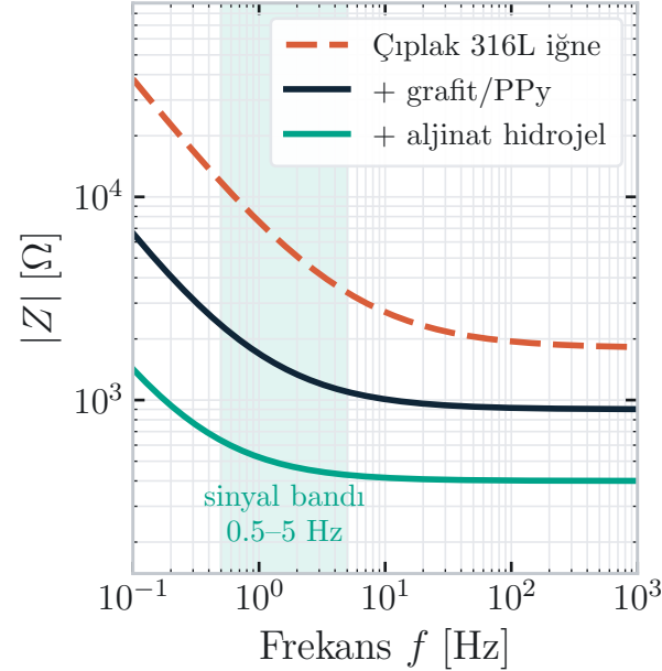
(c) Arayüz empedansı
