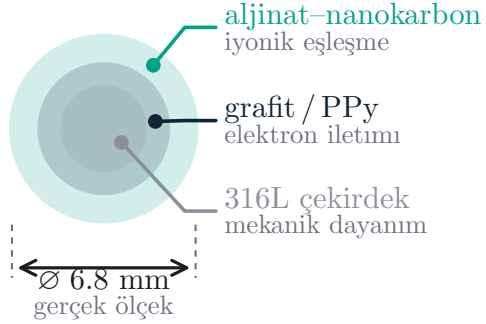
(a) Katman yapısı
