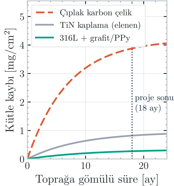
(b) Korozyon dayanımı
