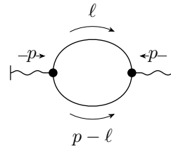
momenta
