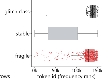
Qwen3-235B-A22B
