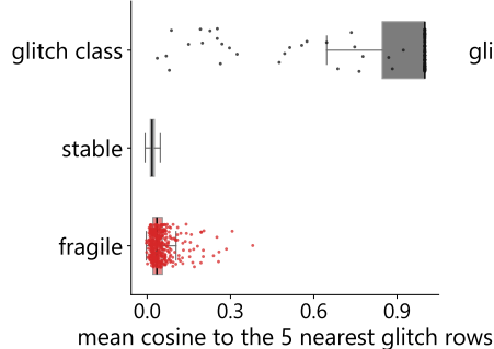
Qwen3-235B-A22B
