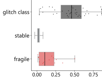
Qwen3-235B-A22B
