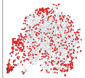
Qwen3-235B-A22B
