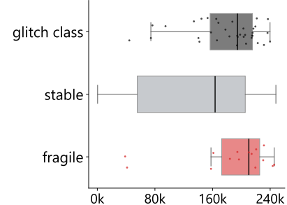
Qwen3-235B-A22B
