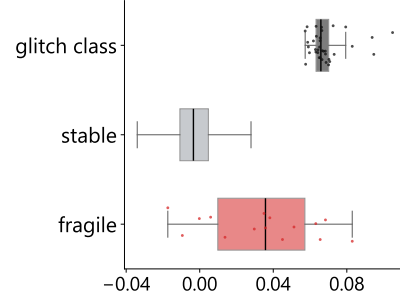
Qwen3-235B-A22B
