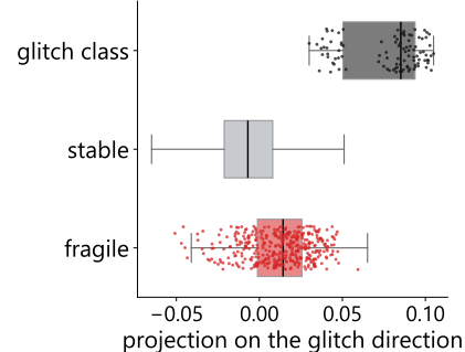
Qwen3-235B-A22B
