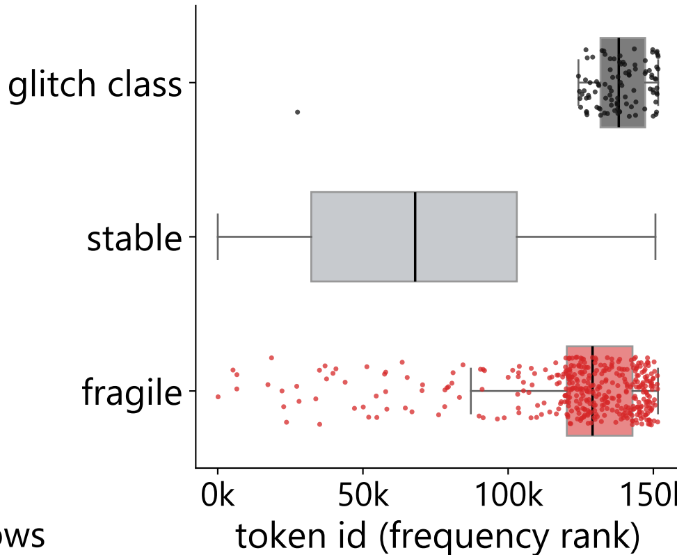
Qwen3-235B-A22B
