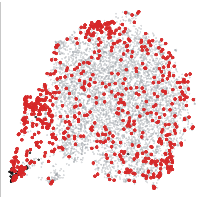
Qwen3-235B-A22B
