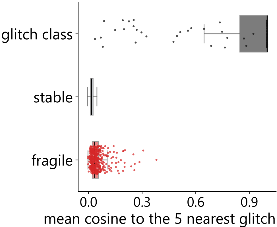
Qwen3-235B-A22B
