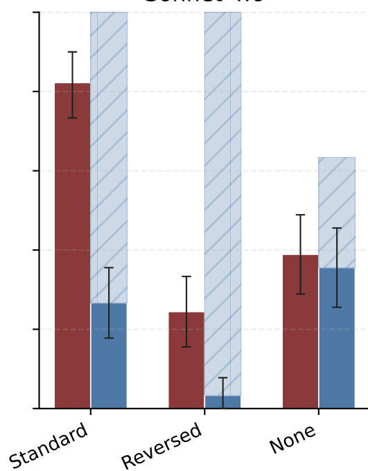
Sonnet 4.6
