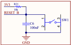
Reset
