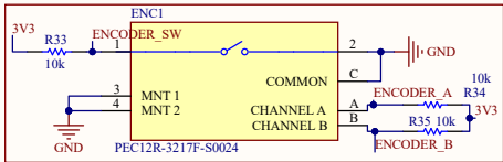
Encoder
