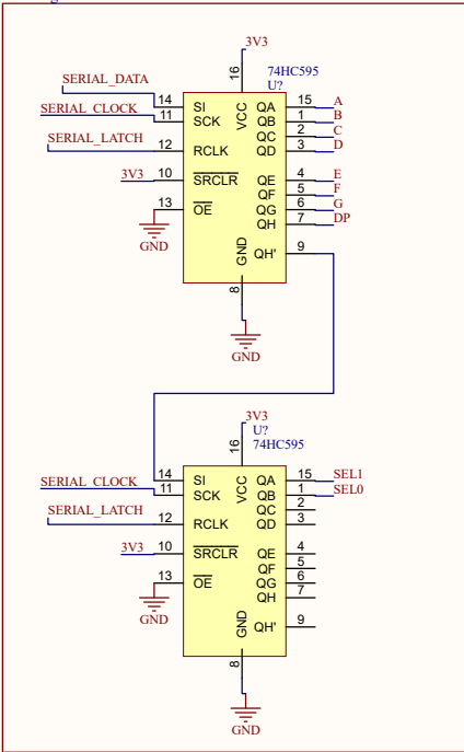
Shift registers
