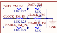
Encoder
