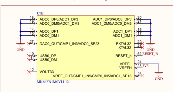
K64F sección analógica
