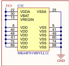
K64F Alimentación
