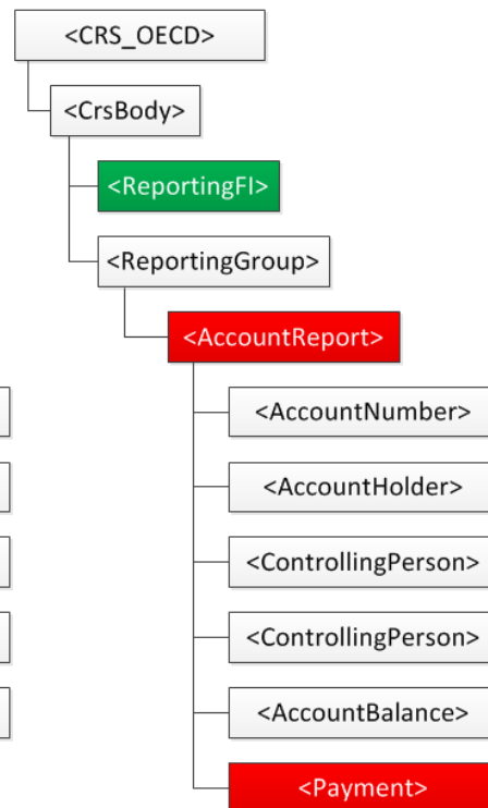
Abbildung 6: Hinzufügen eines Unterelements zu einem AccountReport
