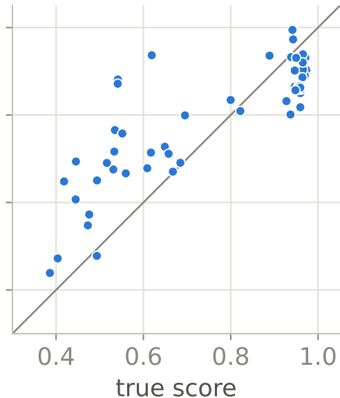
FCN MAE 0.104
