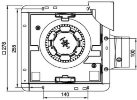
24CHG Dimension
