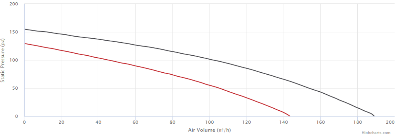
12NSB_220V 60Hz
