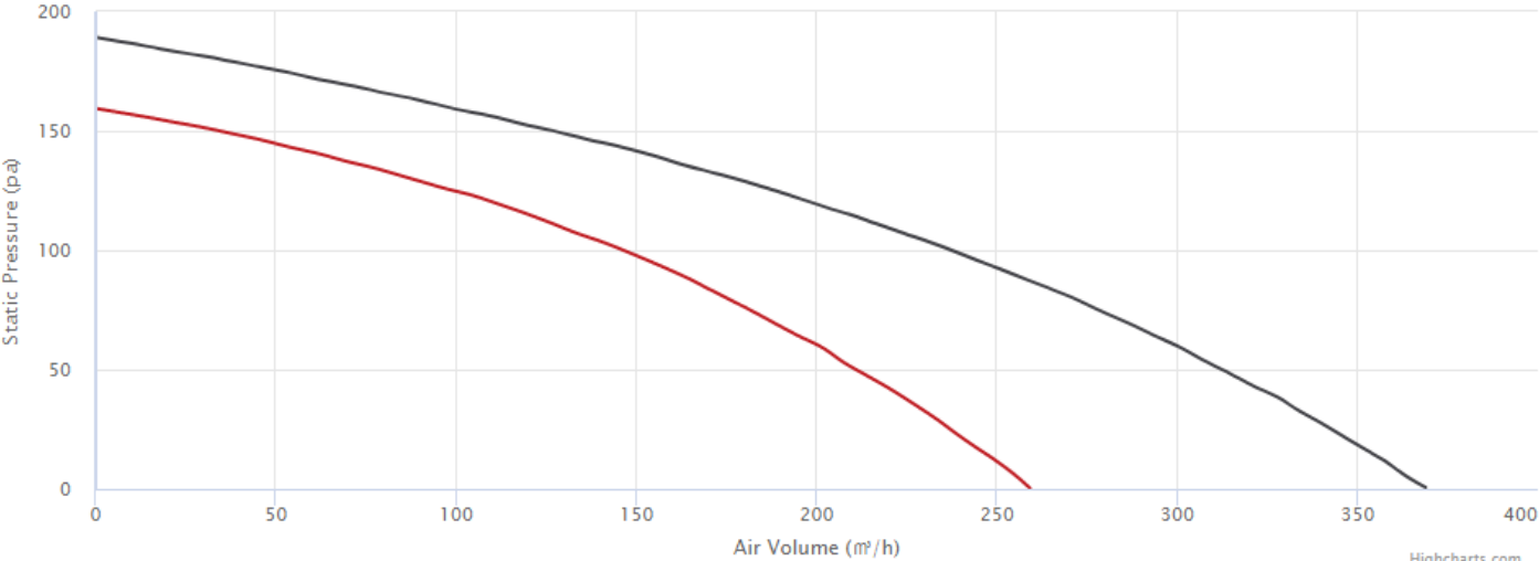
15NSB_220V 60Hz
