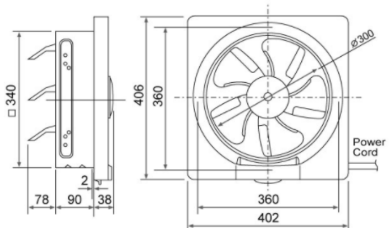
30AUH Dimension
