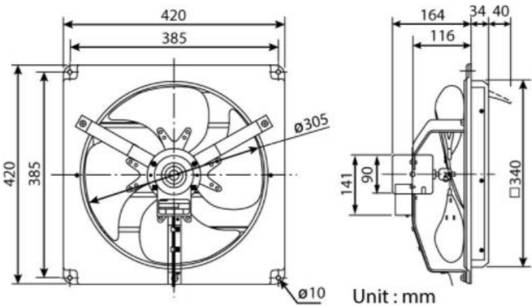
30KQT Dimension
