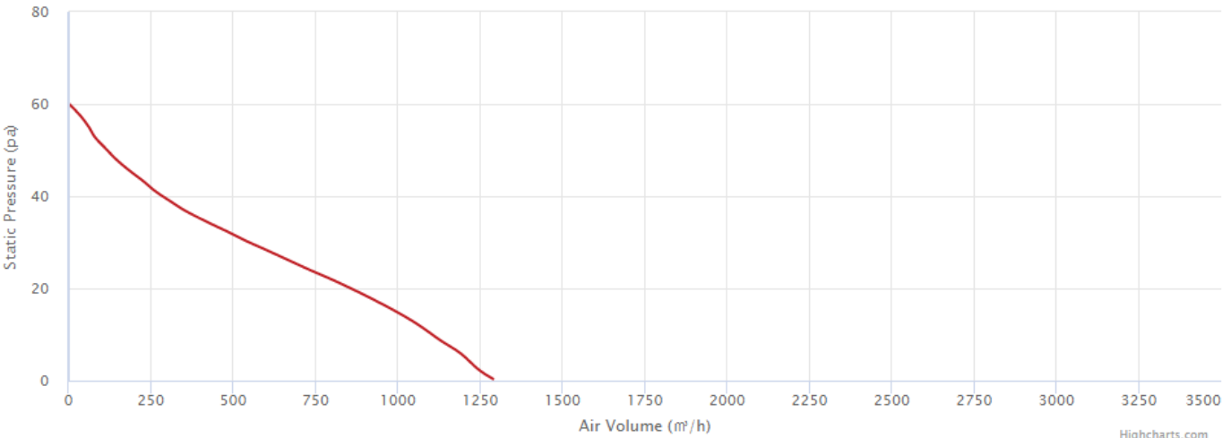
30KQT_220V 60Hz
