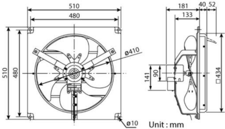
40KQT Dimension
