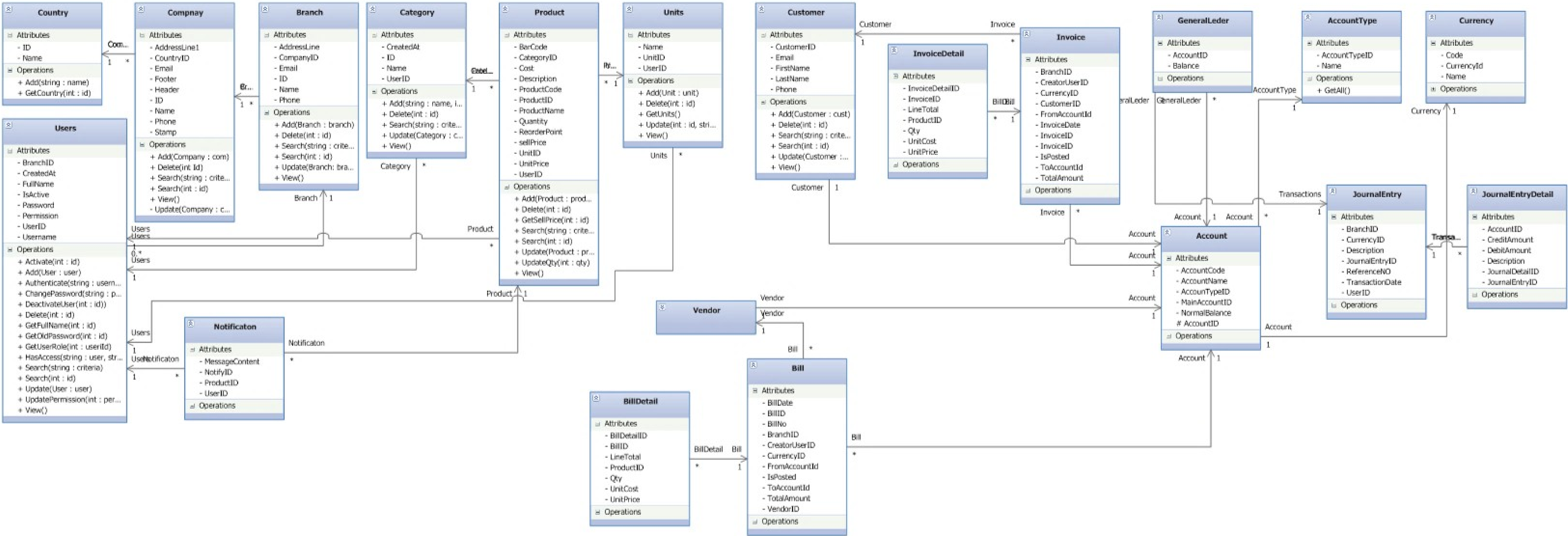
cd UMLClassDiagram2
