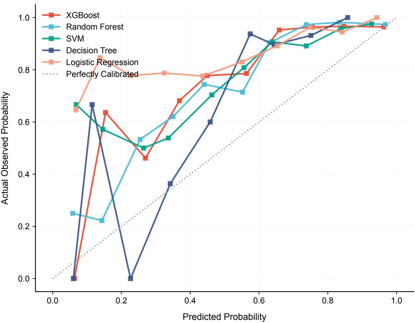
External Calibration: COMPOSITE (subgroup_no_renal = 0)
