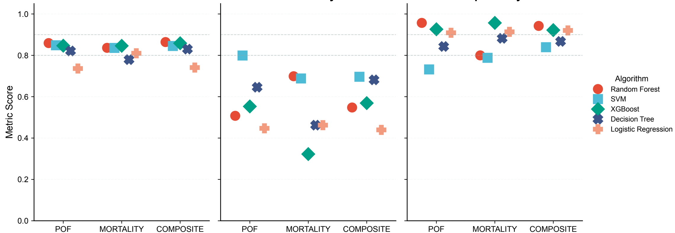
AUC
