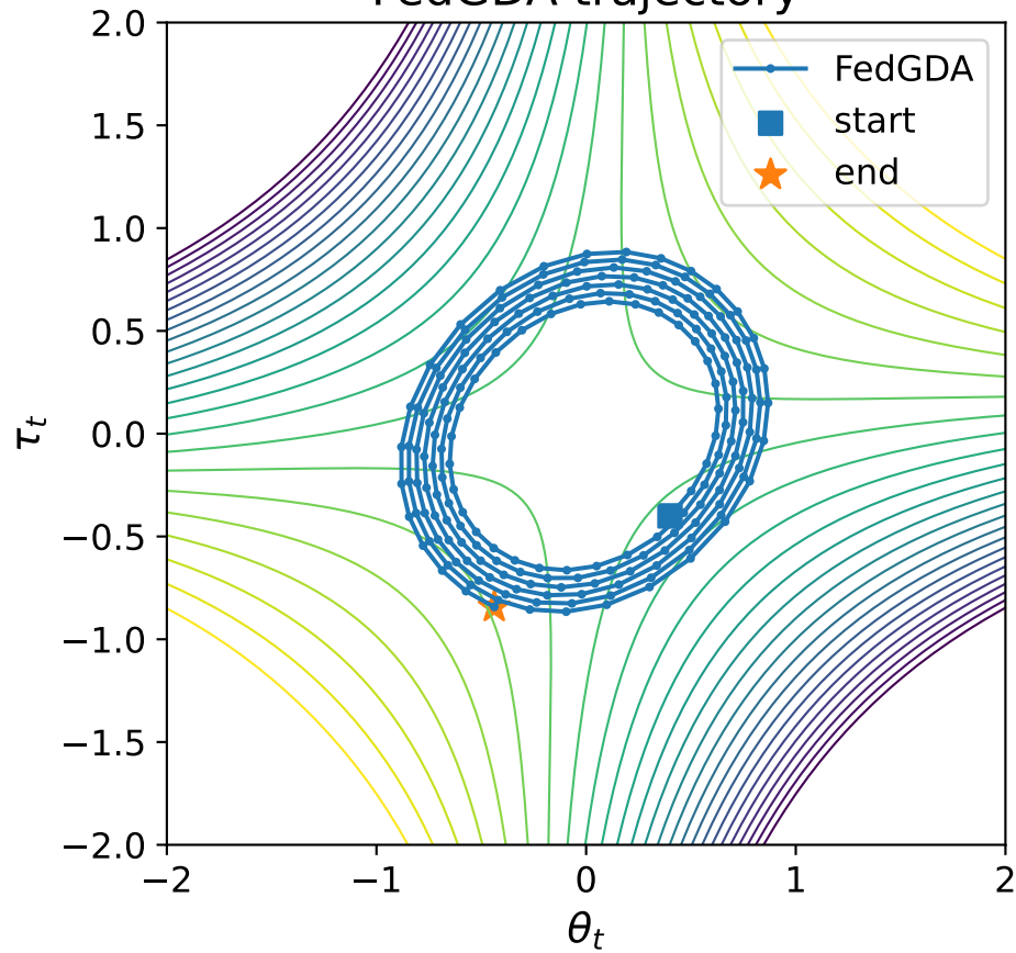
FedGDA trajectory
