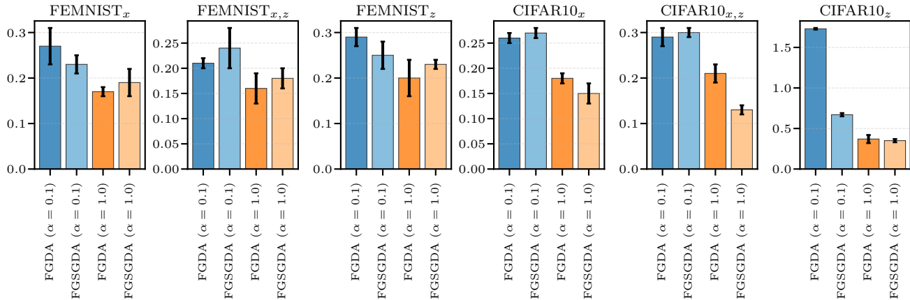
Test MSE
