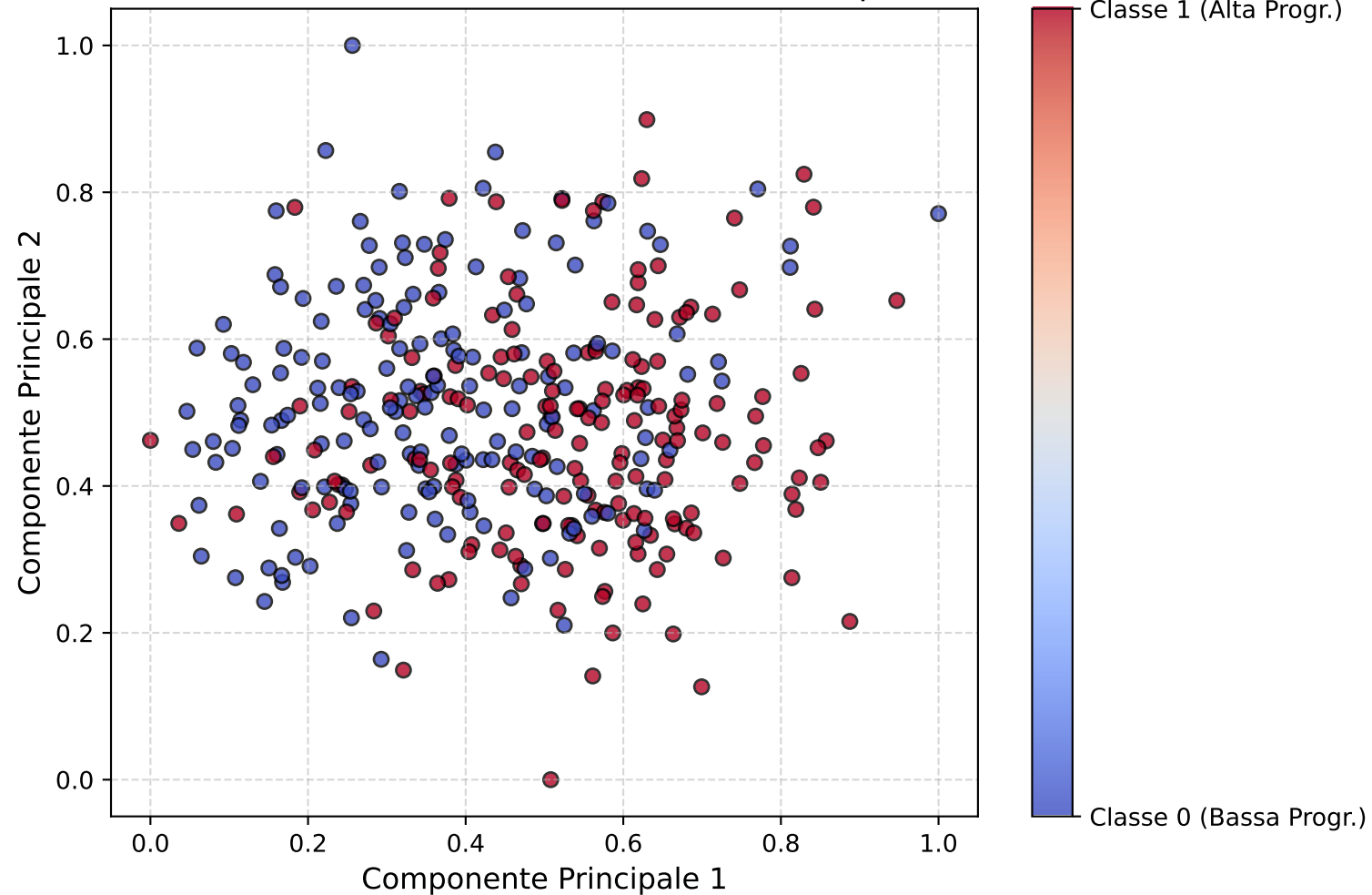
Distribuzione delle Classi (PCA - Prime 2 Componenti)
