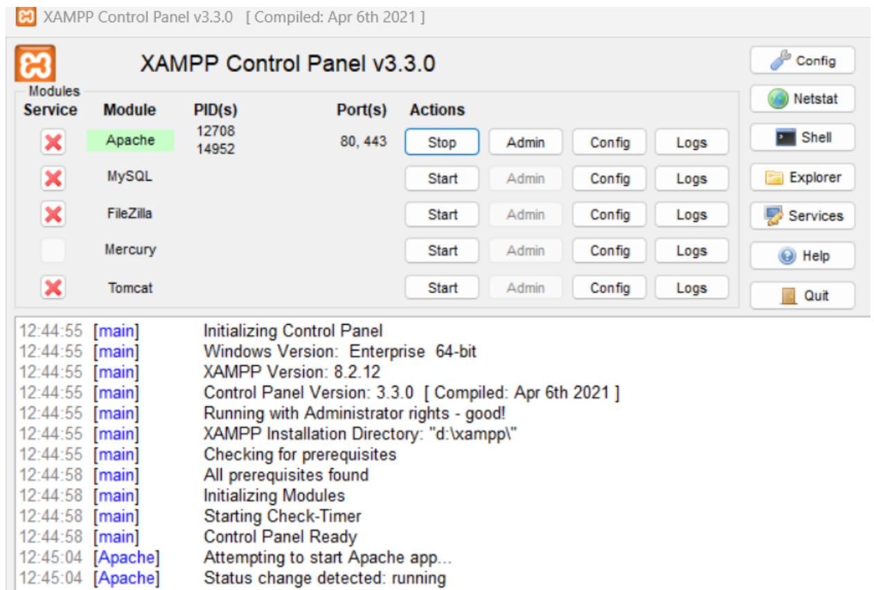
Рисунок 1 — Запуск Apache
