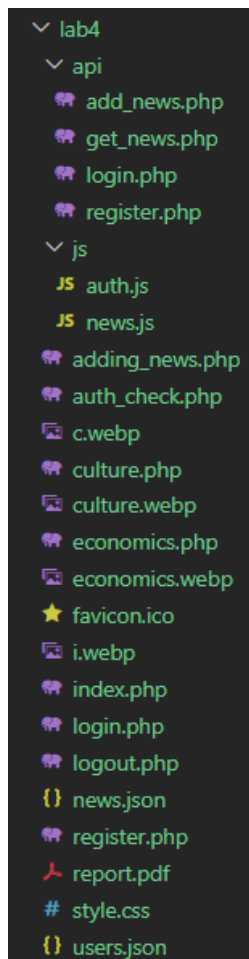
Рисунок 1 – Структура проекта
