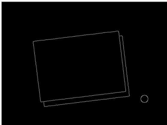
Canny, пороги 42/104
