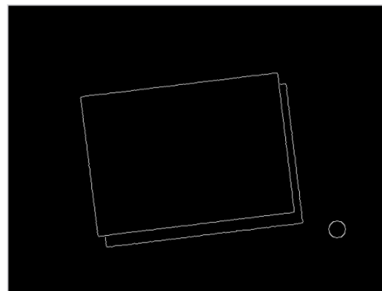
Canny F1 = 1.00
