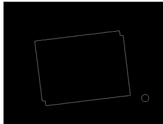
RETR_EXTERNAL: 2 контуров
