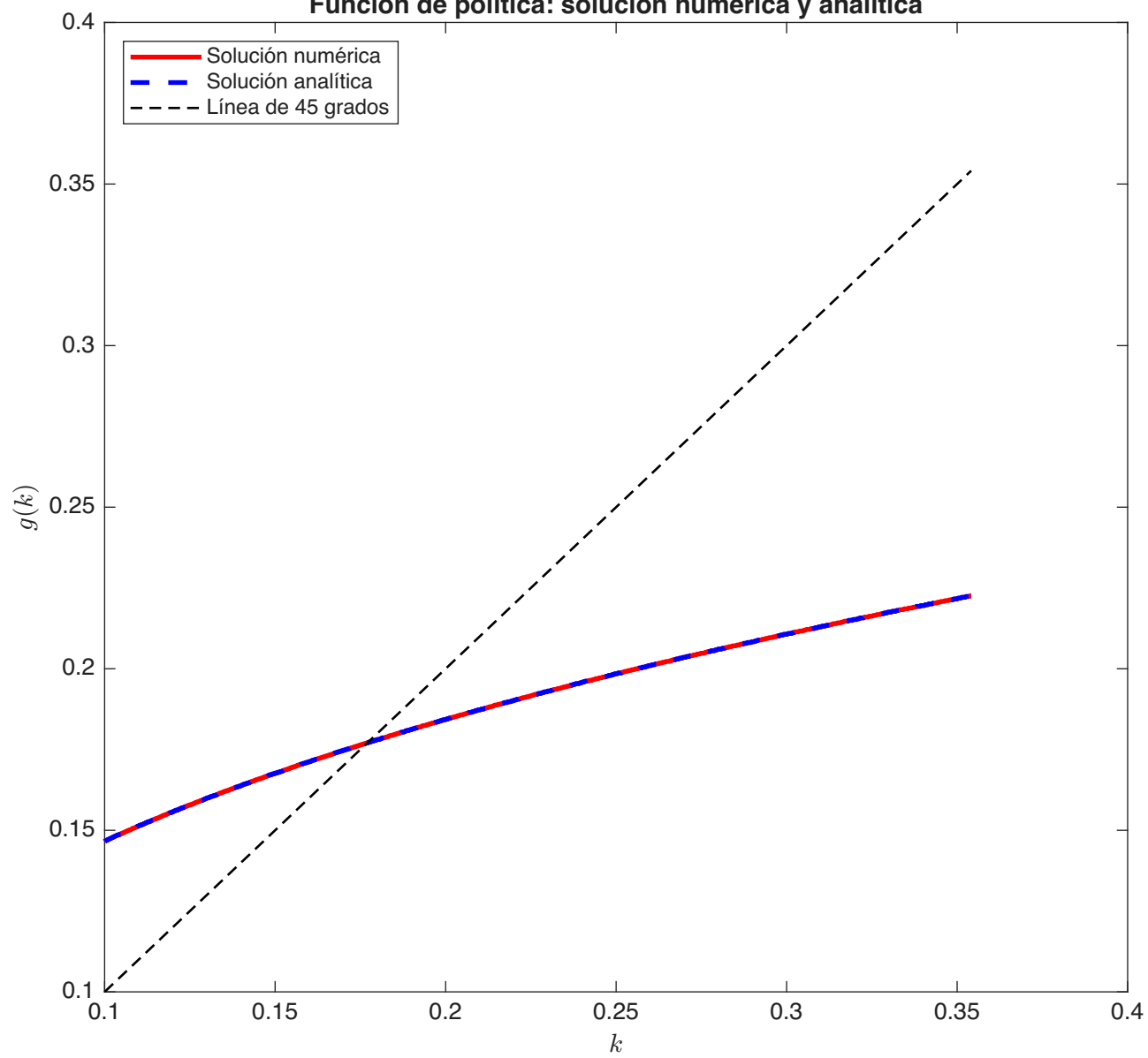
Función de política: solución numérica y analítica
