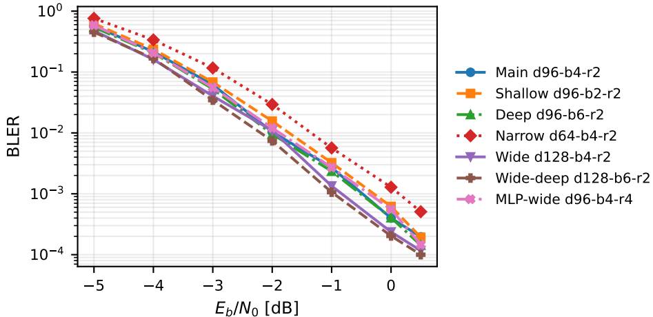
U3: UPAIR ablation
