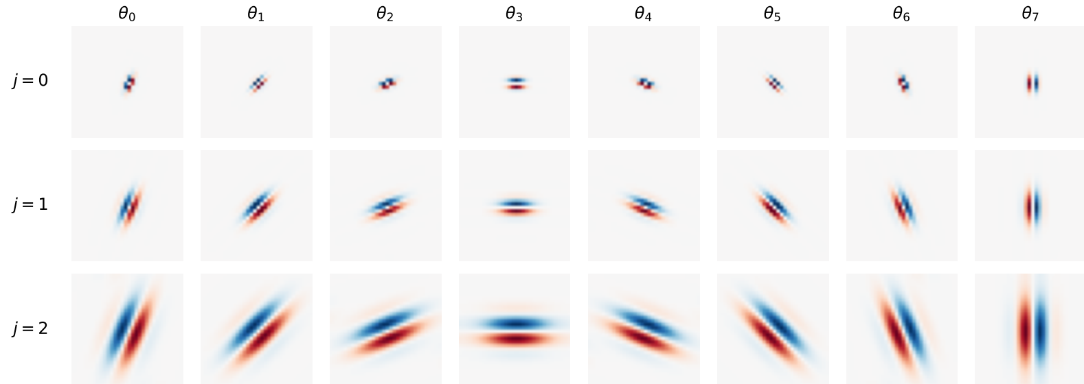
Banco de wavelets de Morlet (parte imaginaria), J = 3 , L = 8
