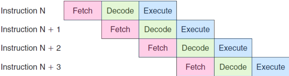
图 6.1 Cortex-M3 的三级流水线
