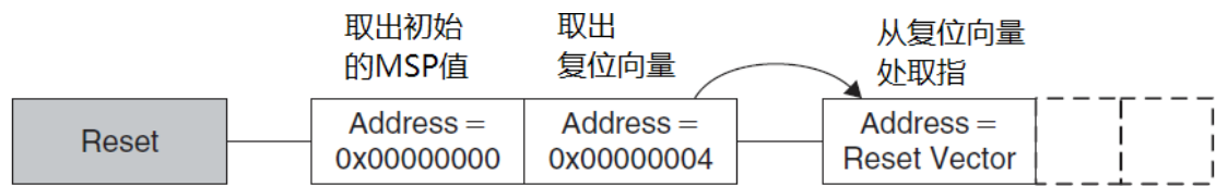
图 3.17 复位序列
