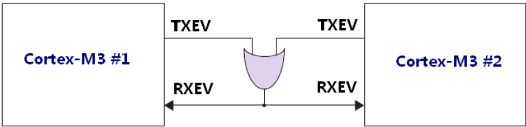
图 13.4 双核处理系统间的事件信号连接
