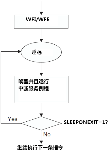
图 13.3 SleepOnExit 功能演示
