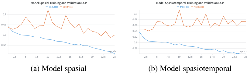
Gambar 4.7 Kurva training loss dan validation loss pada eksperimen learning rate 5e-4 : (a) model spasial dan (b) model spasiotemporal.
