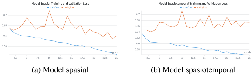
Gambar 4.7 Kurva training loss dan validation loss pada eksperimen learning rate 5e-4: (a) model spasial dan (b) model spatiotemporal.
