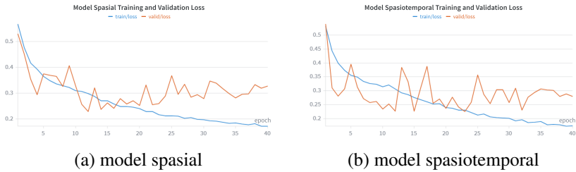
Gambar 4.6 Kurva training loss dan validation loss pada eksperimen epoch maksimum 40: (a) model spasial dan (b) model spasiotemporal.
