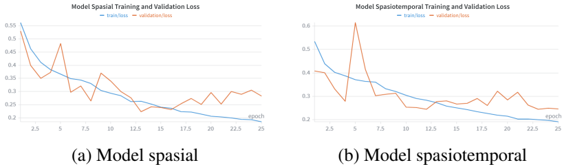
Gambar 4.3 Kurva training loss dan validation loss pada eksperimen baseline .
