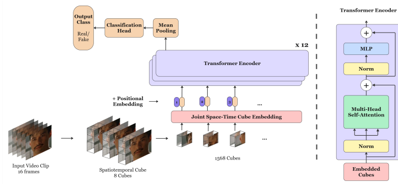
Gambar 3.10 Arsitektur model spatiotemporal berbasis VideoMAE untuk klasifikasi deepfake
