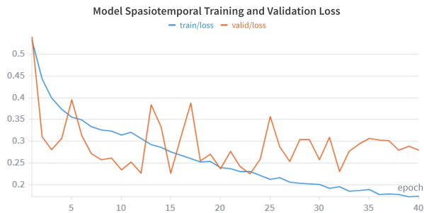
(b) Model spasiotemporal
