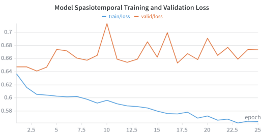
(b) Model spasiotemporal
