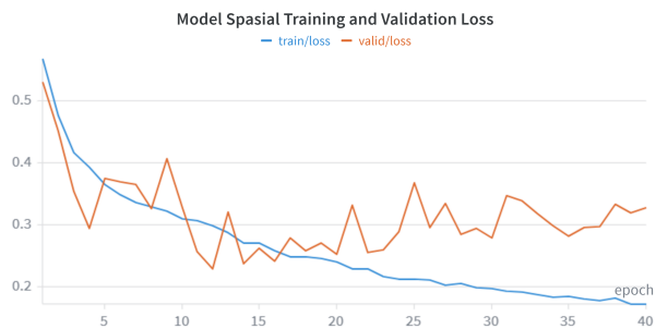
Gambar 4.5 Kurva training loss dan validation loss pada eksperimen epoch maksimum 40 untuk model spasial.
