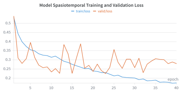
Gambar 4.6 Kurva training loss dan validation loss pada eksperimen epoch maksimum 40 untuk model spasiotemporal.
