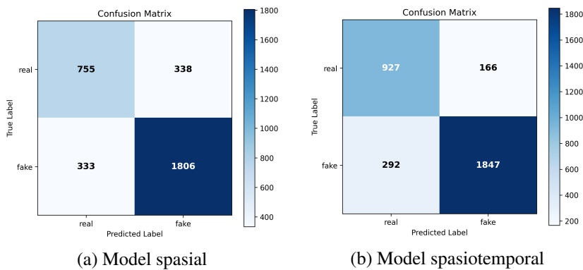
Gambar 4.4 Confusion matrix pada eksperimen baseline .
