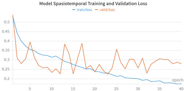
Gambar 4.8 Kurva training loss dan validation loss pada eksperimen epoch maksimum 40 untuk model spatiotemporal.
