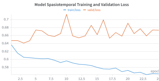
Gambar 4.10 Kurva training loss dan validation loss pada eksperimen learning rate 5e-4 untuk model spasiotemporal.
